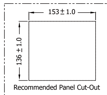
前視圖 (面板開孔)
