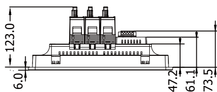
上視圖
