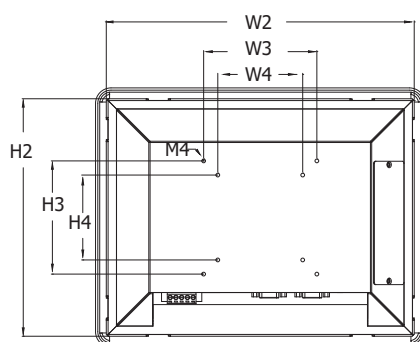
後視圖
