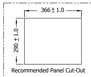
前視圖 (面板開孔)
