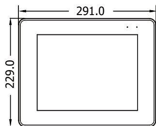
前視圖
