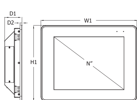
左視圖
