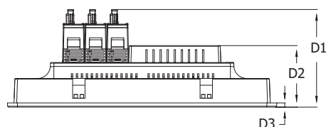
上視圖
