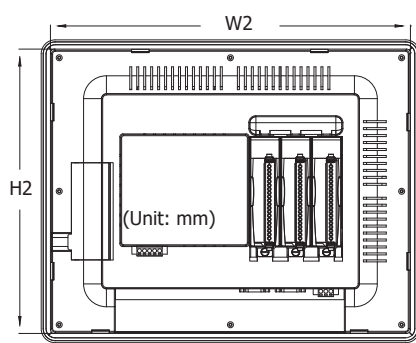
後視圖
