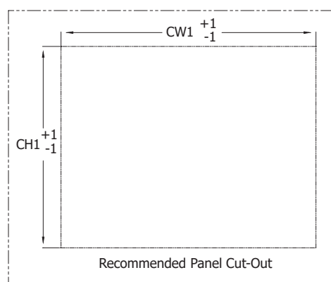
前視圖 (面板開孔)
