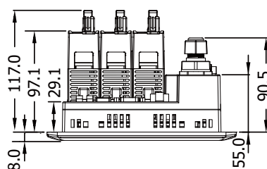
上視圖
