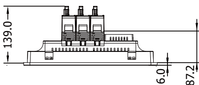
上視圖
