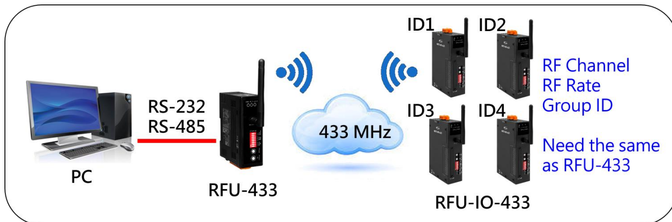
電腦透過一個 RFU-433 控制站號 1 ~ 4 的 RFU-IO-433 模組
