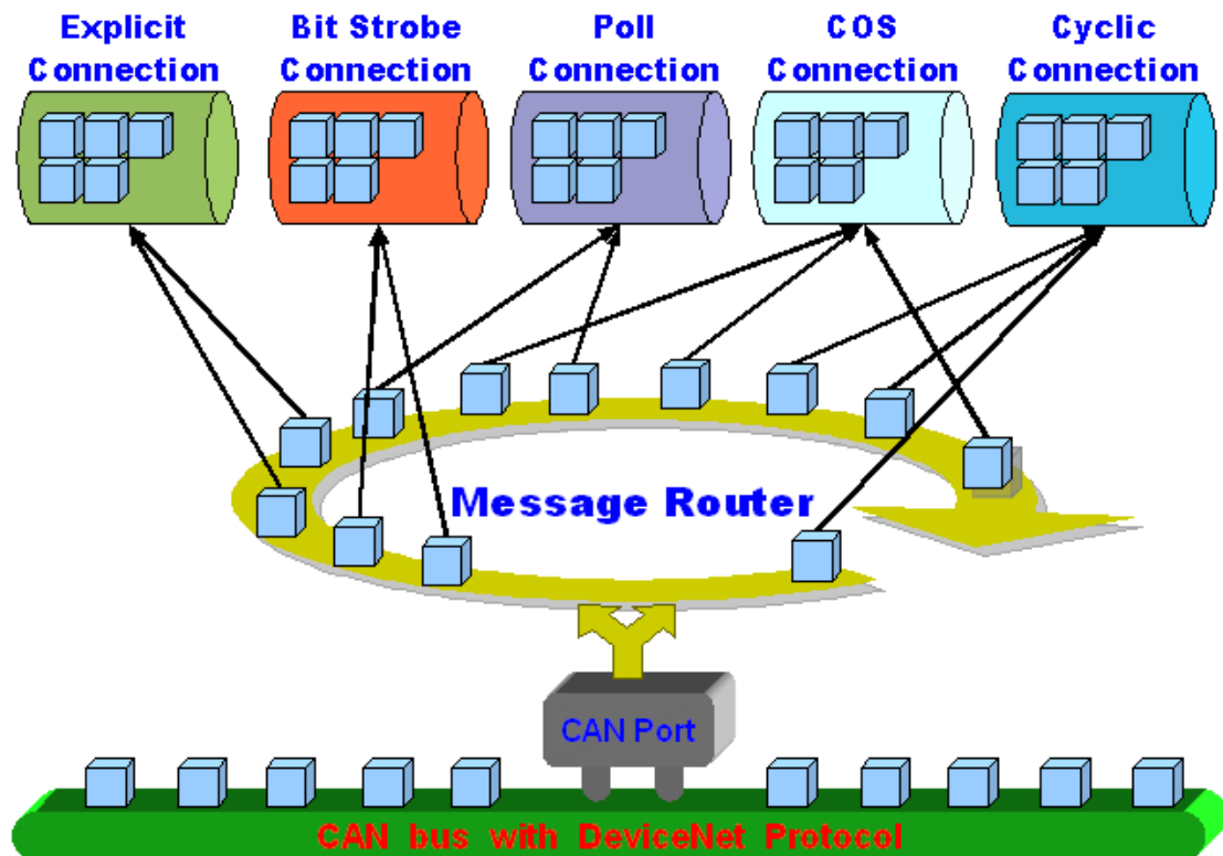
圖 1.6 信息路由器
