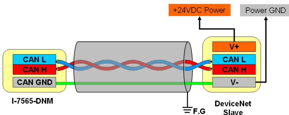
圖 2.6 帶有 24V 直流電源的 CAN 總線連接
