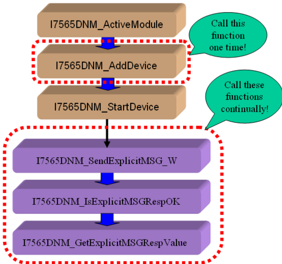
圖 3.9 “SendExplicitMSG_W” 流程圖
