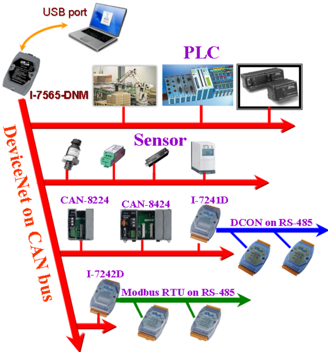
圖 1.3 應用架構
