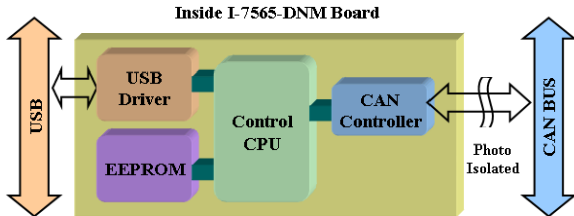
圖 1.8 I-7565-DNM 模組方塊圖
