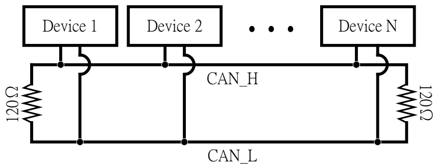
圖 2.4 CAN 總線網路拓撲結構
