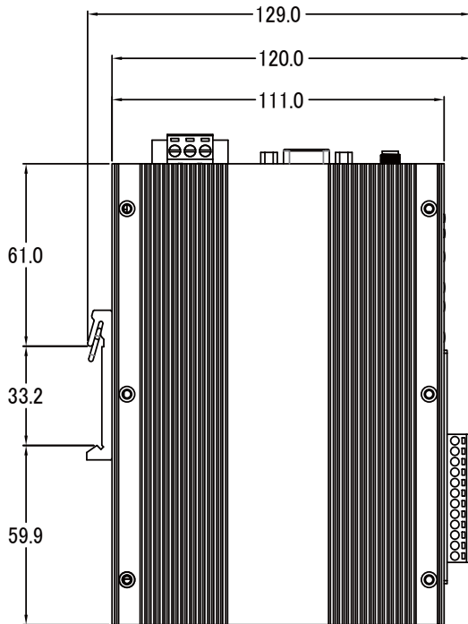
左視圖
