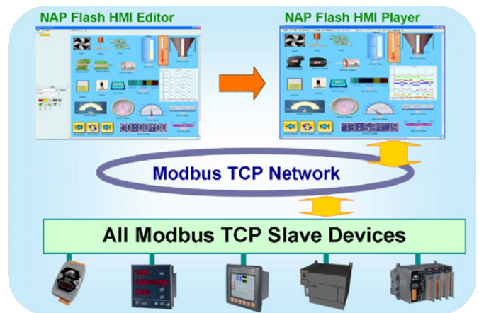
▲ NAP Flash HMI Tools 系統架構
