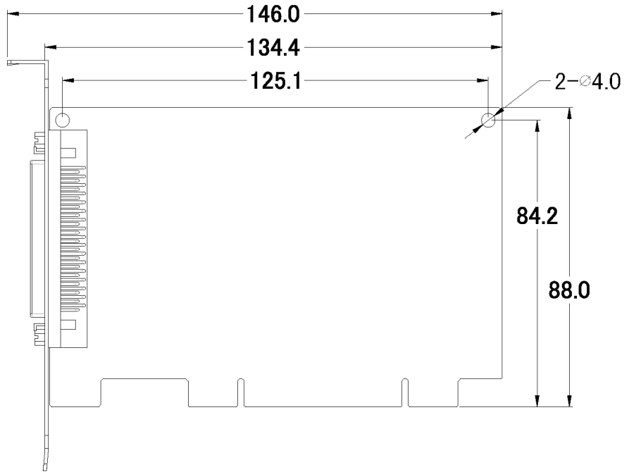
前視圖
