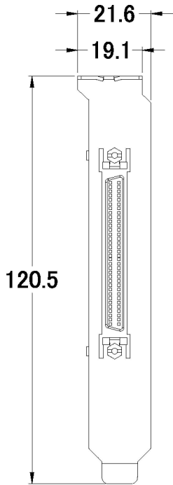
左視圖
