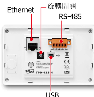
TPD-433-H 後視圖
