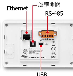
TPD-433-H-EU 後視圖
