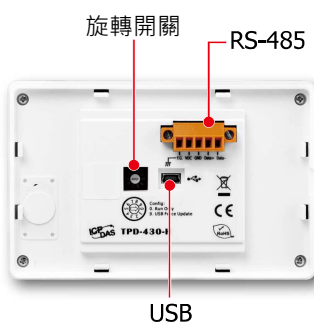
TPD-430-H 後視圖
