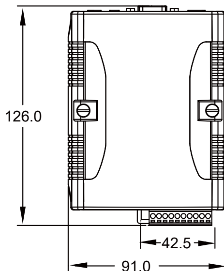
前視圖
