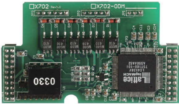
X702 2-axis 編碼器模組
