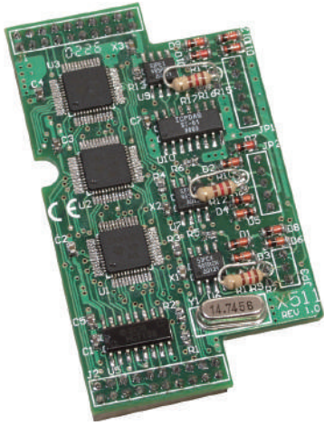
X511 3 埠 RS-485
