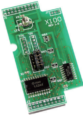
X100 8 通道數位輸入
