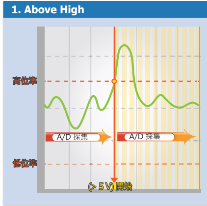
1. Above High: 訊號高於高位準時觸發
