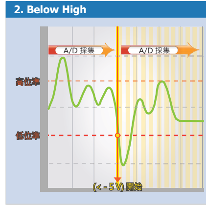
2. Below Low: 訊號低於低位準時觸發
