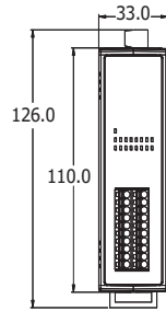
前視圖
