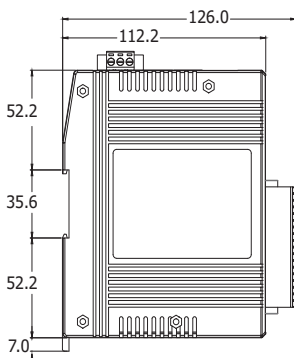
左側視圖
