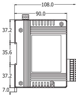
左側視圖
