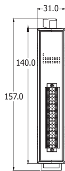
前視圖
