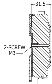
剖視圖
