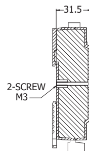
剖視圖
