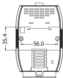
後視圖
