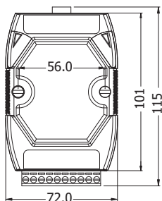
前視圖
