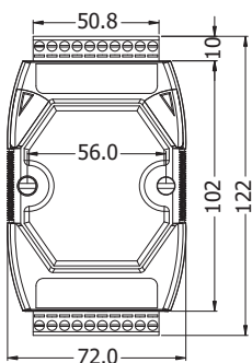
前視圖
