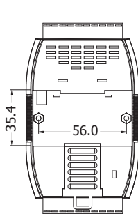
後視圖
