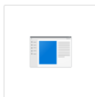
ua-am335x_1.4.2.0_app.tar
