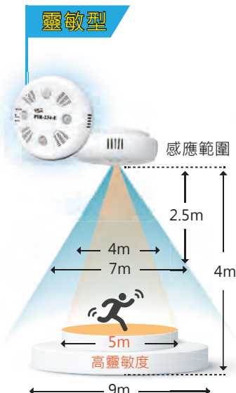
PIR-234-E PIR-234-WF
