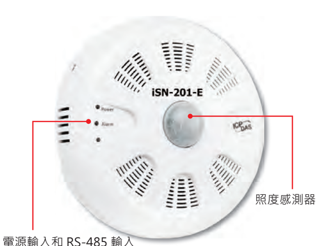
iSN-201-E
