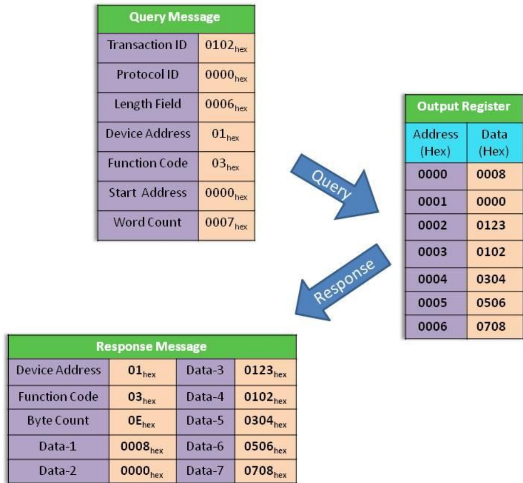
圖 7-3: 使用 Modbus TCP 命令(功能碼 03 hex ) 讀取傳送的 CAN 訊息格式
