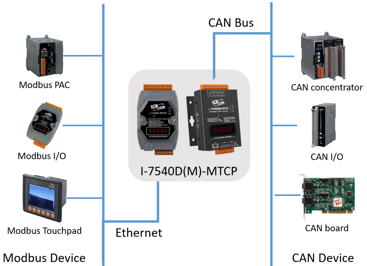
圖 1-1: I-7540D(M)-MTCP Modbus TCP 模式的應用
