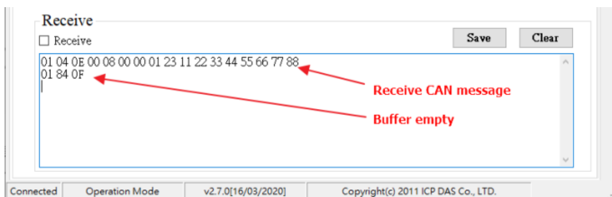
圖 5-2: I-7540D(M)-MTCP Modbus 模式傳回的 CAN 訊息
