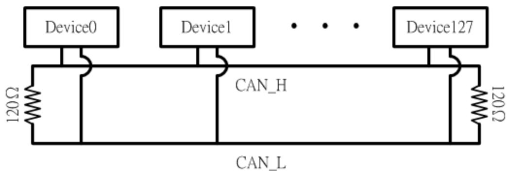
圖 2-4: 終端電阻
