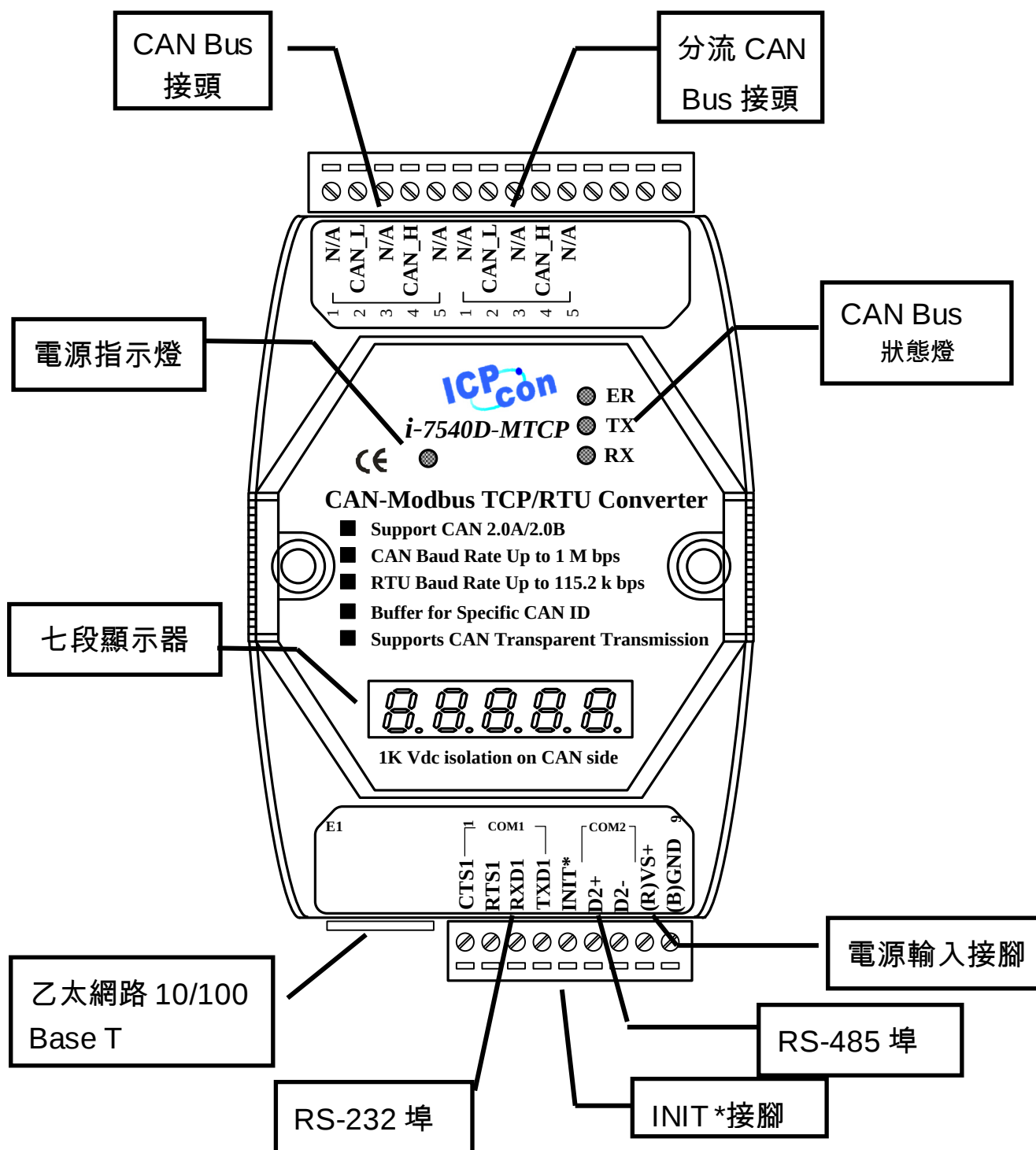
圖 2-2: I-7540D(M)-MTCP 腳位定義
