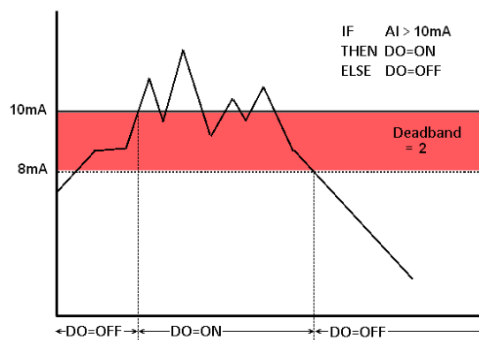
圖 7-22: AI Deadband 示意圖(作用於大於條件)
