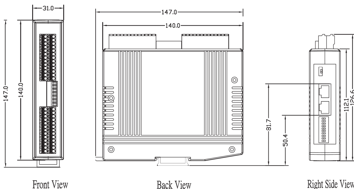
圖1-1 MN-3253的產品外觀
