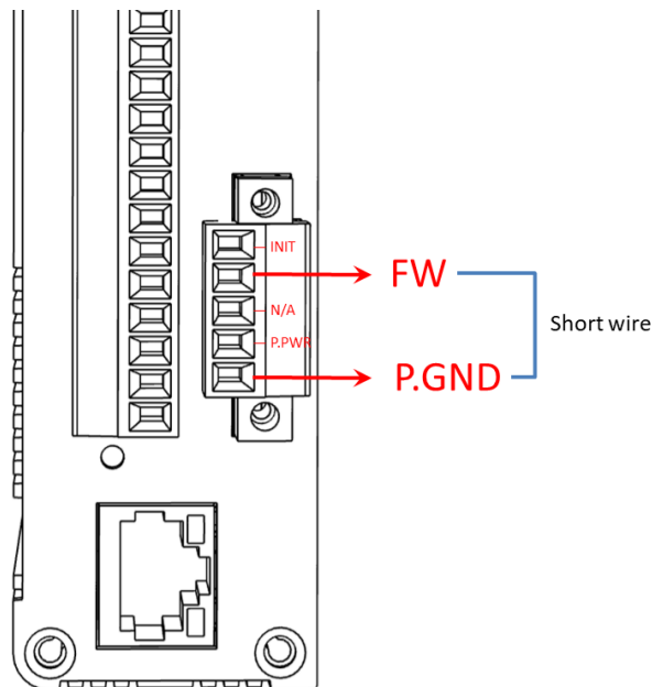
圖 11. BNET-2107M 的「FW」與「GND」腳短接
