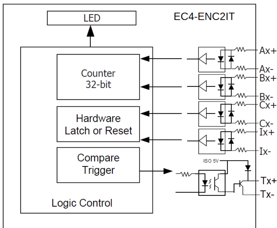
圖 5: DIO 線路
