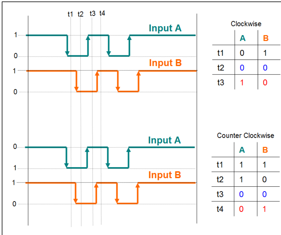
圖 30: 輸入信號"A"極性改變, 反轉計數方向
