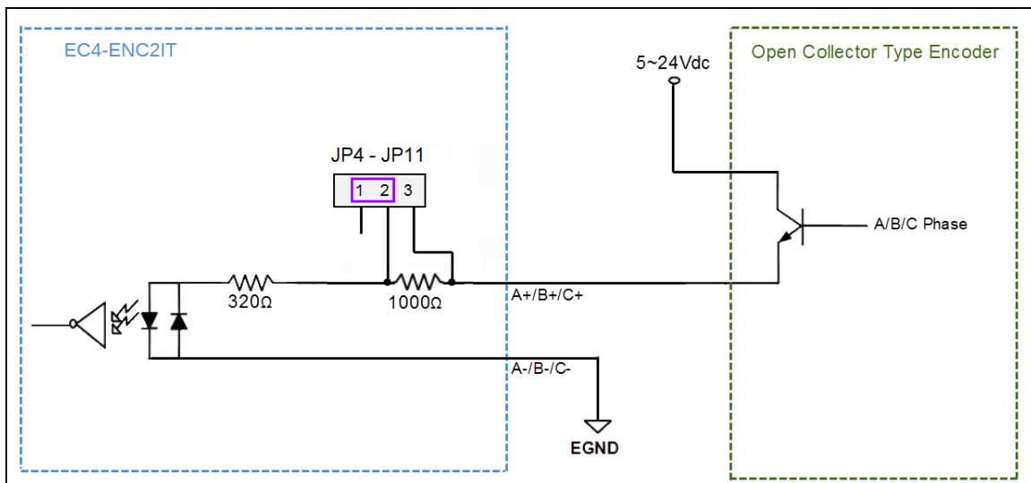
圖 8: 開路集極接線圖 (Sink DI)
