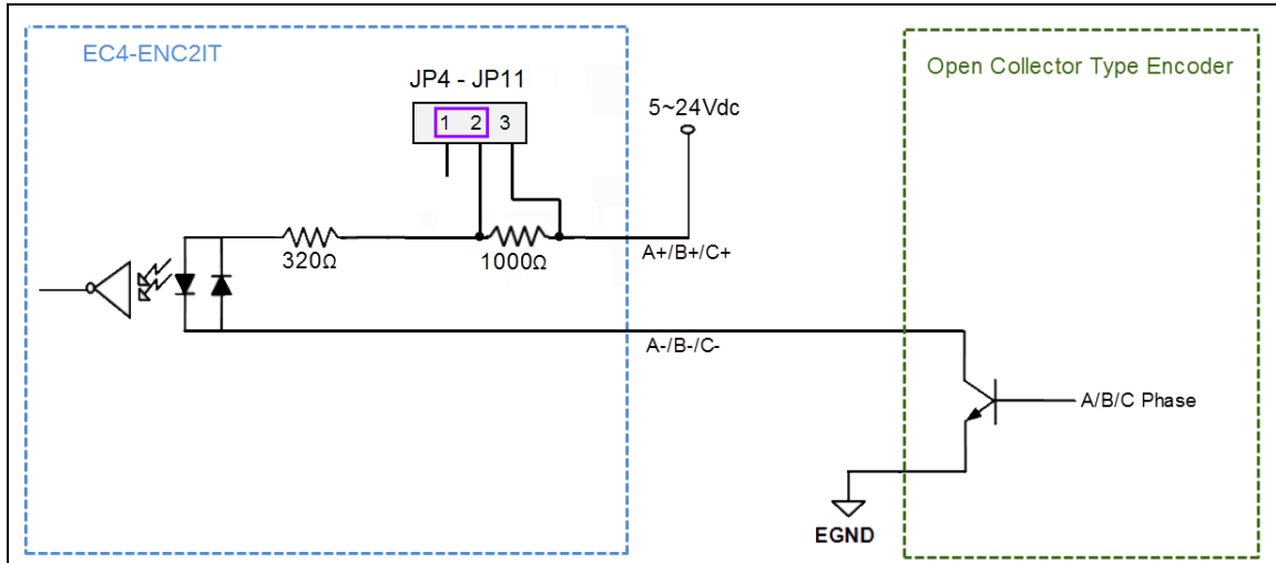
圖 7: 開路集極接線圖 (Source DI)
