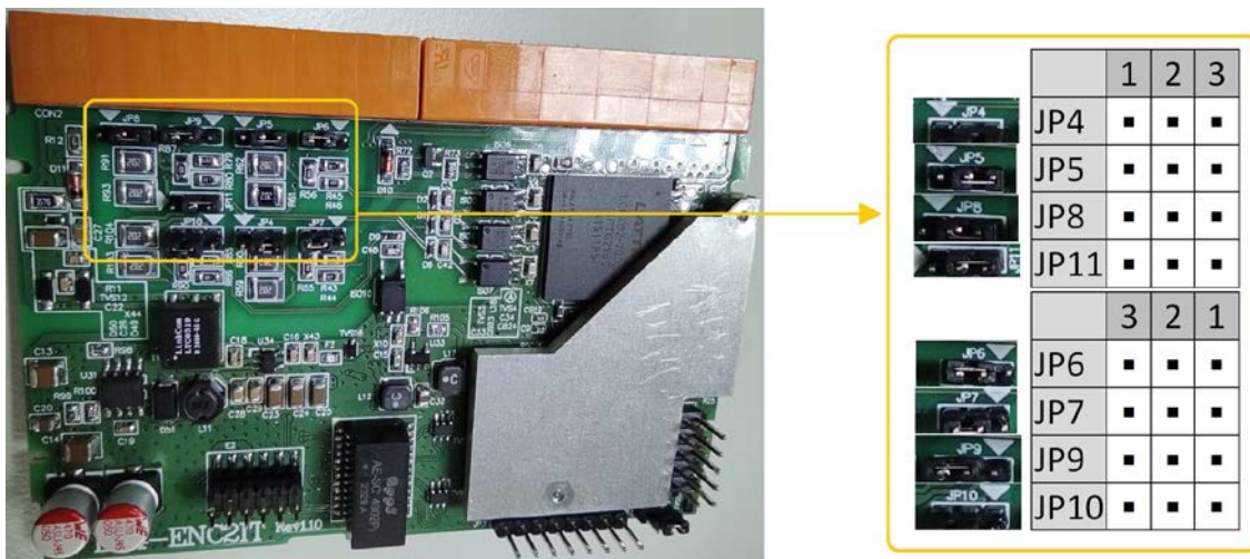
圖 9: 跨接器位置
