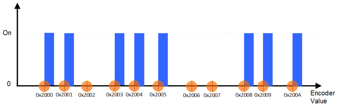
圖 32: 通道 0 的陣列比較位置
