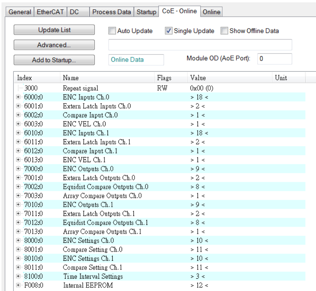
圖 40: "CoE - Online " 標籤頁
