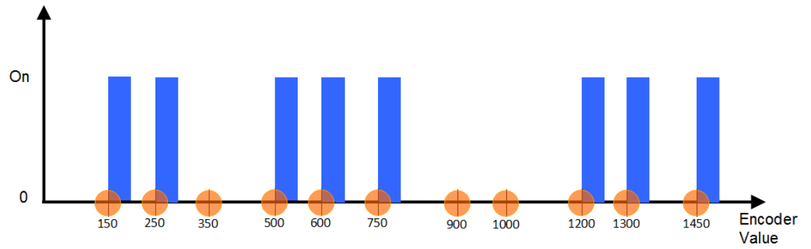
圖 37:比較位置與其 DO 觸發設定
