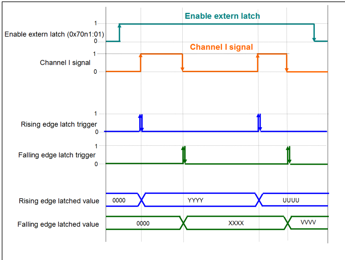
圖 31:上升緣與下降緣鎖存
