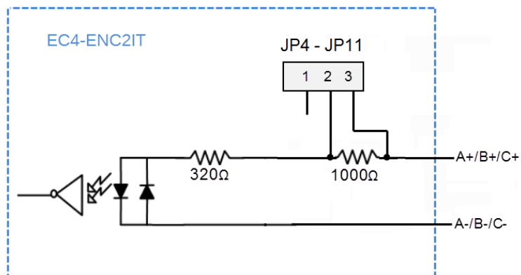
圖 6: 編碼器通道線路
