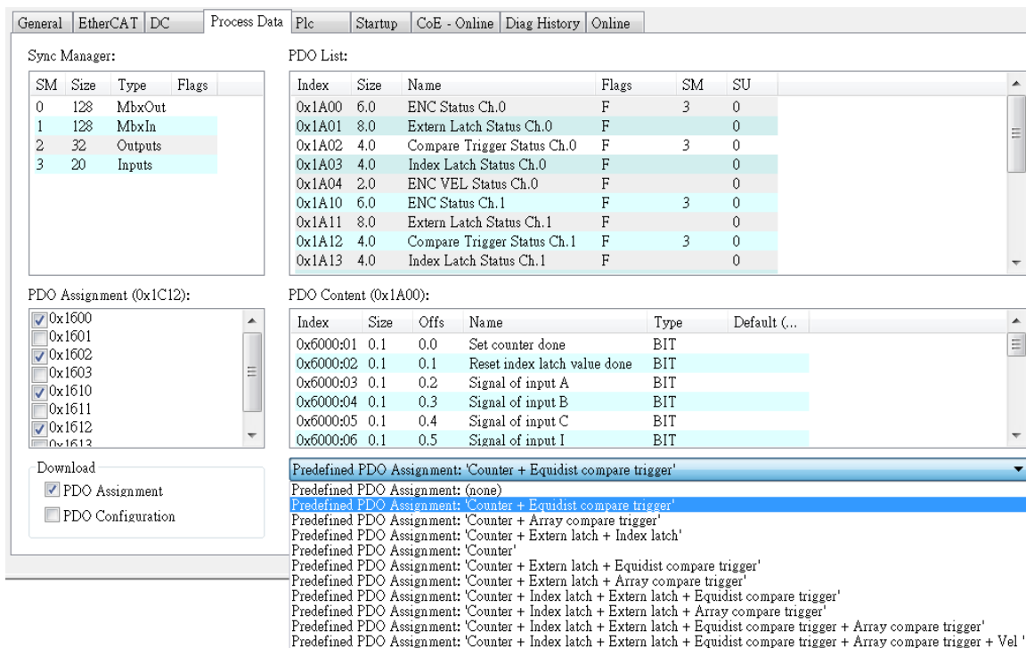
圖 23: 預定義的 PDO 分配選擇
