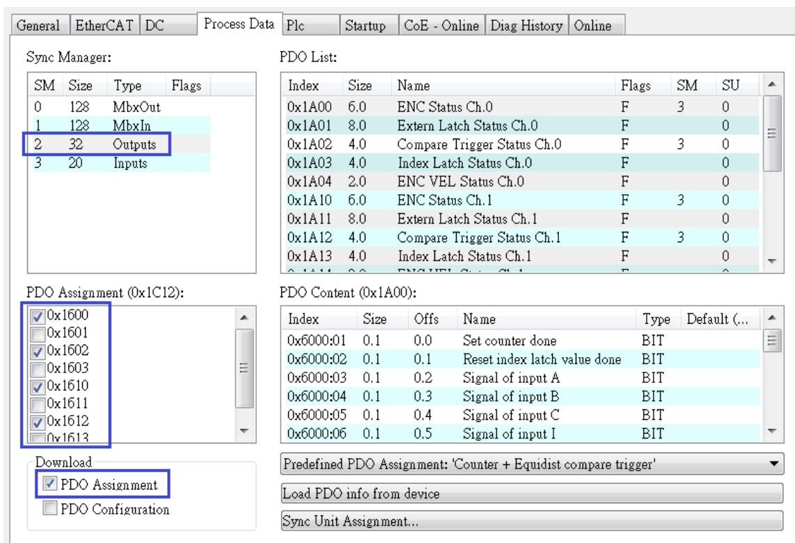
圖 24: 預定義 PDO 分配選擇
