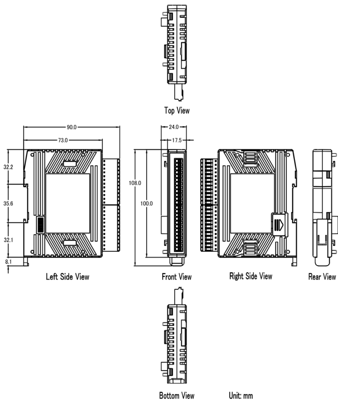
圖 1: EC4-ENC2IT 外型尺寸
