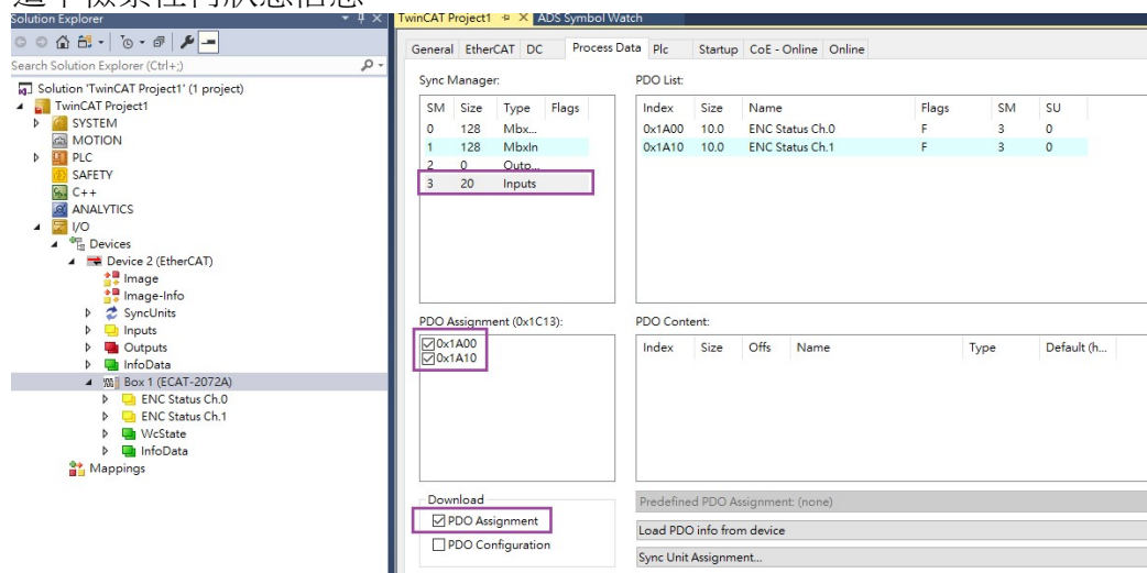
圖 19: Predefined PDO assignment 選項
