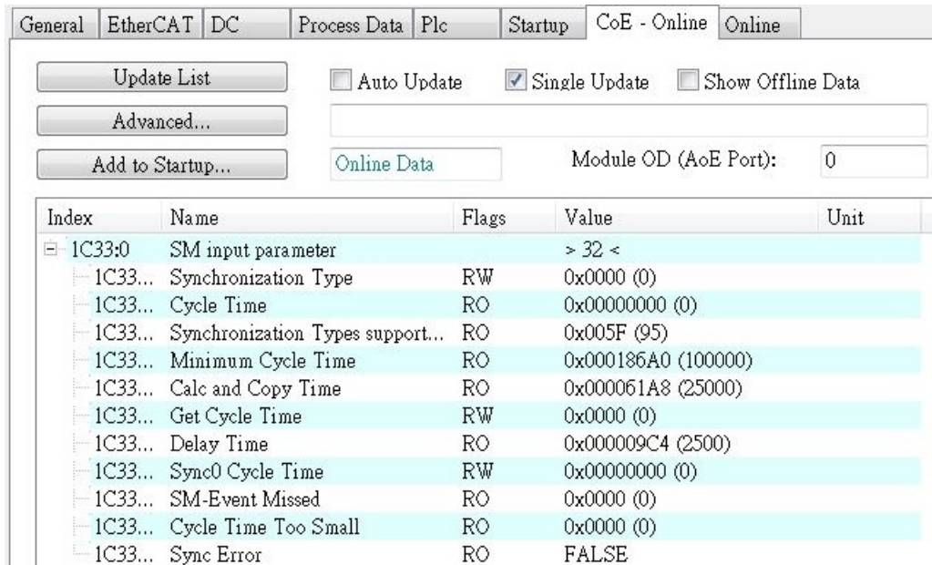
圖 12: 自由運行模式的 SyncManager 設定
