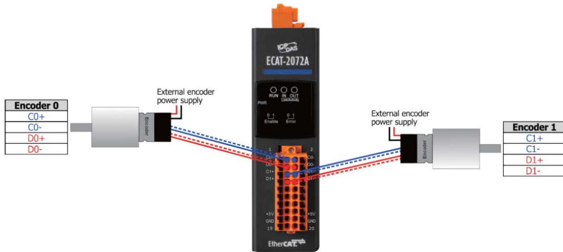
圖 7: ECAT-2072A 編碼器連接
