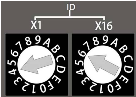
圖 4: ECAT-2074A 別名旋鈕
