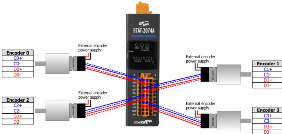
圖 7: ECAT-2074A 編碼器連接
