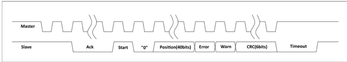
圖 22: BiSS-C 模式(單向)
