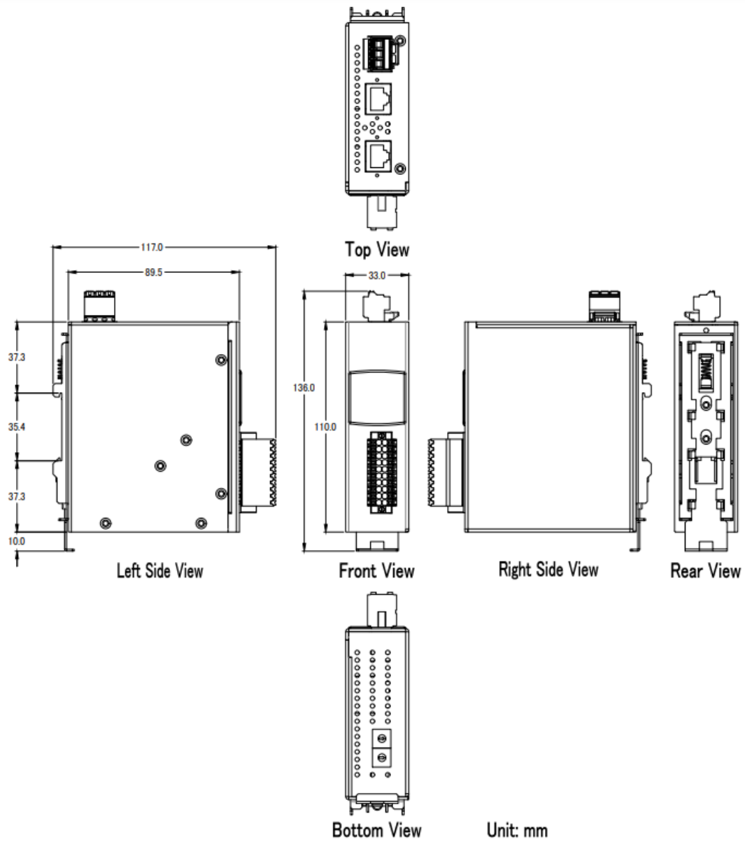
圖 1: ECAT-2074A 外型尺寸
