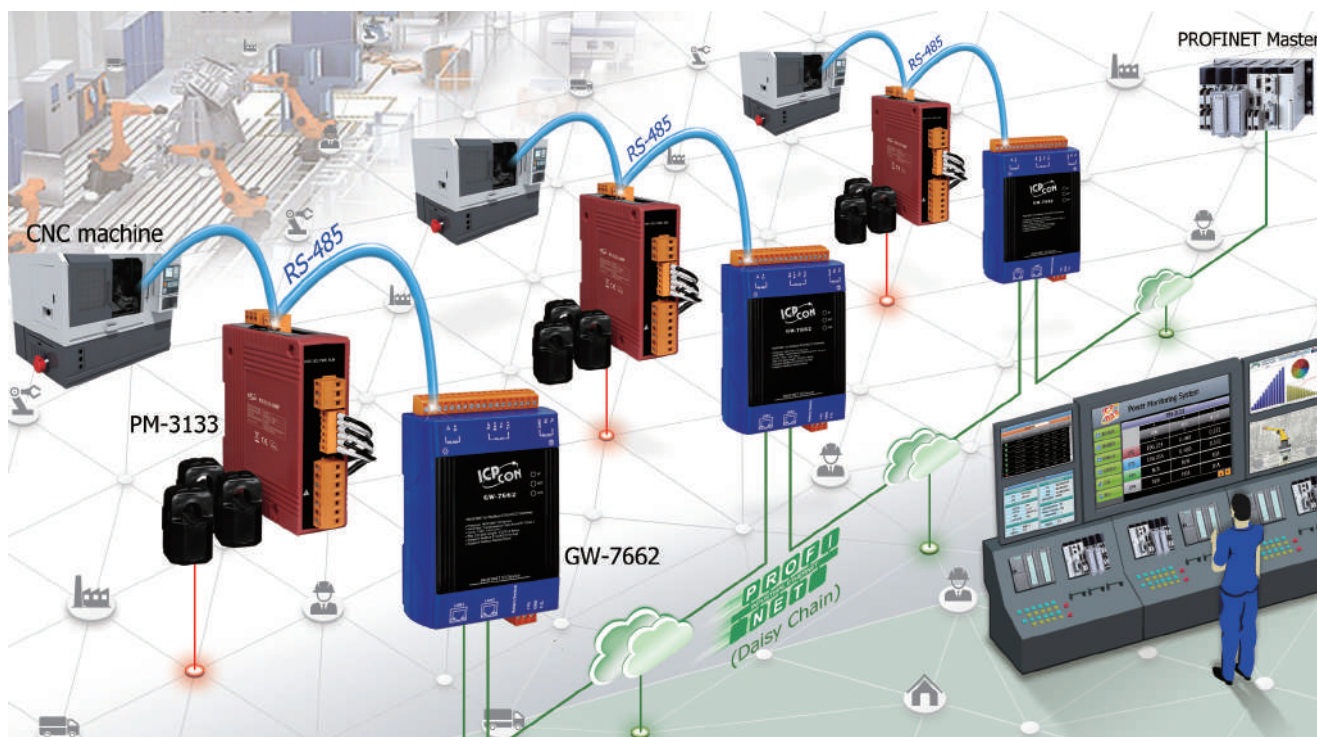
▲透過 PROFINET 的快速傳輸，可迅速取得所有設備的電力資訊
