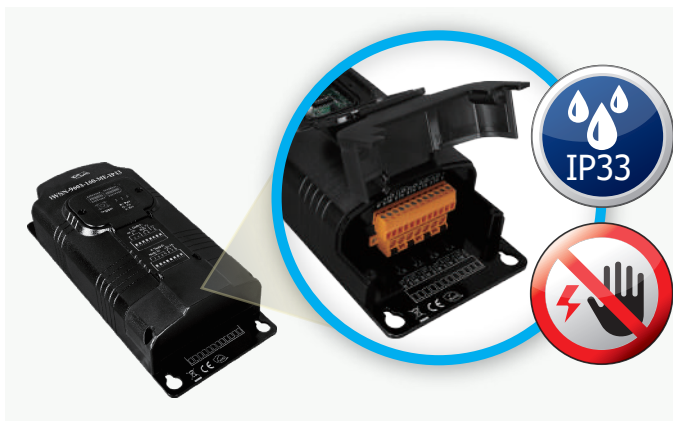
IP33 異物及水氣預防機構設計
