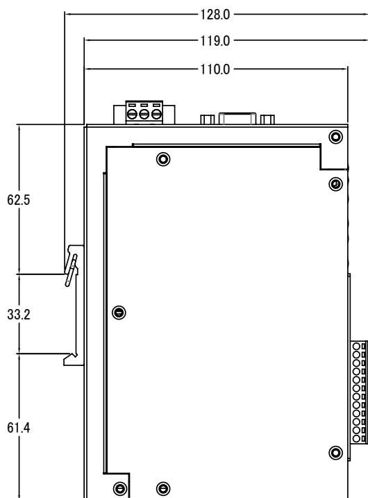
左視圖
