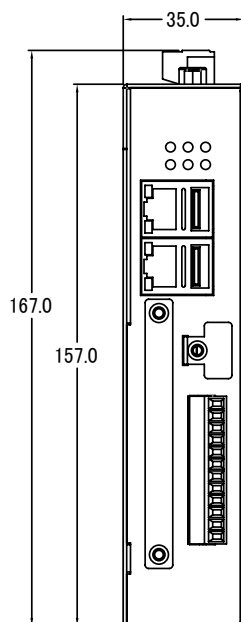
前視圖
