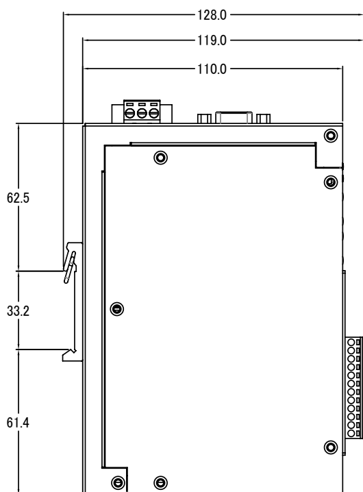
左視圖
