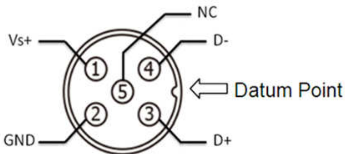
Power & RS-485
