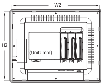
後視圖
