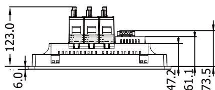
上視圖
