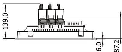
上視圖
