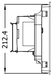
左視圖
