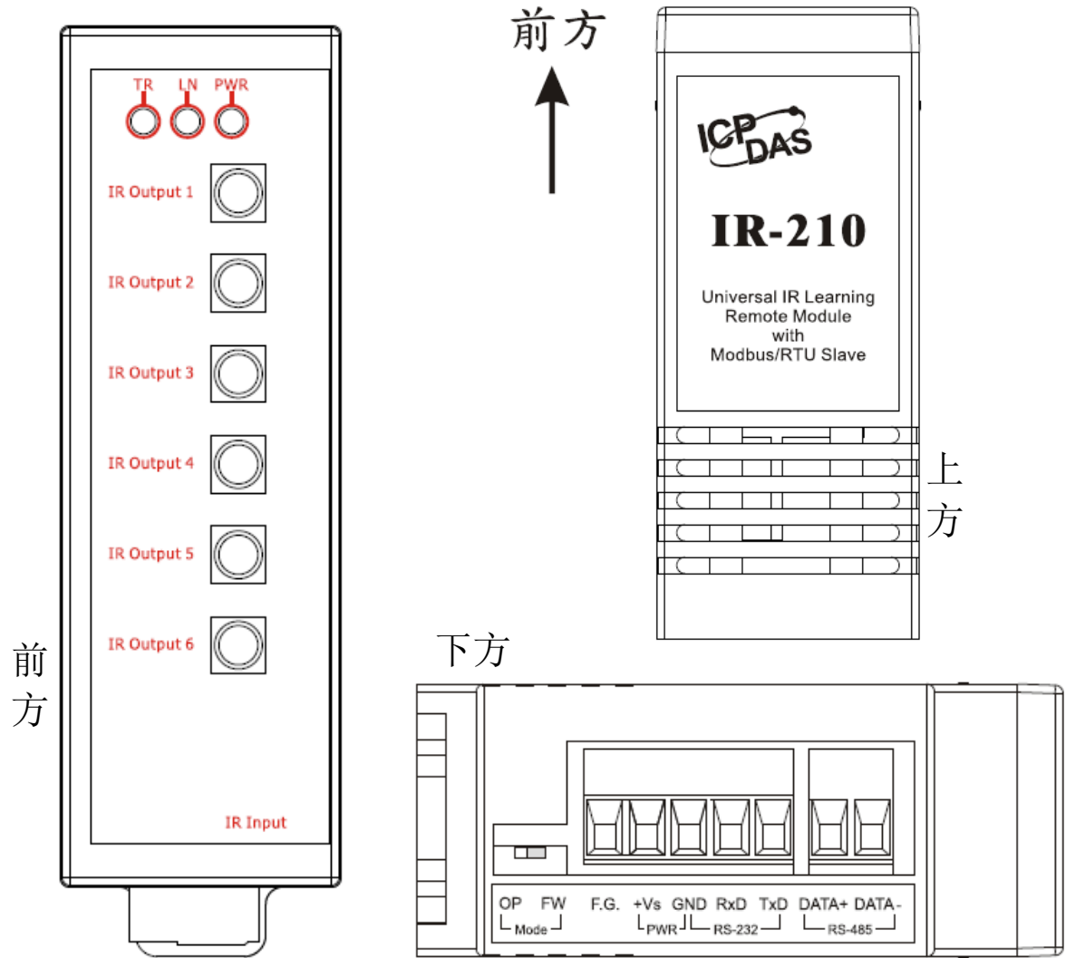
图 2-1、IR-210 产品外观 (前方/上方/下方)
