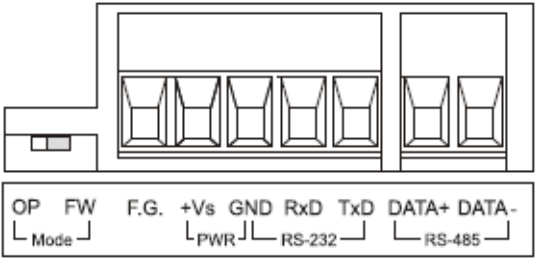
图 2-3、IR-210 螺丝端子台
