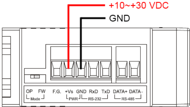
图 2-10、电源接线图
