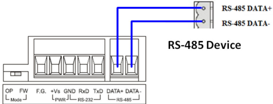
图 2-7、RS-485 联机
