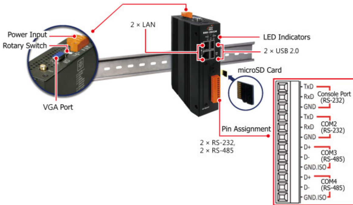
圖 1-6 BRK-2841M 機構圖(1)
