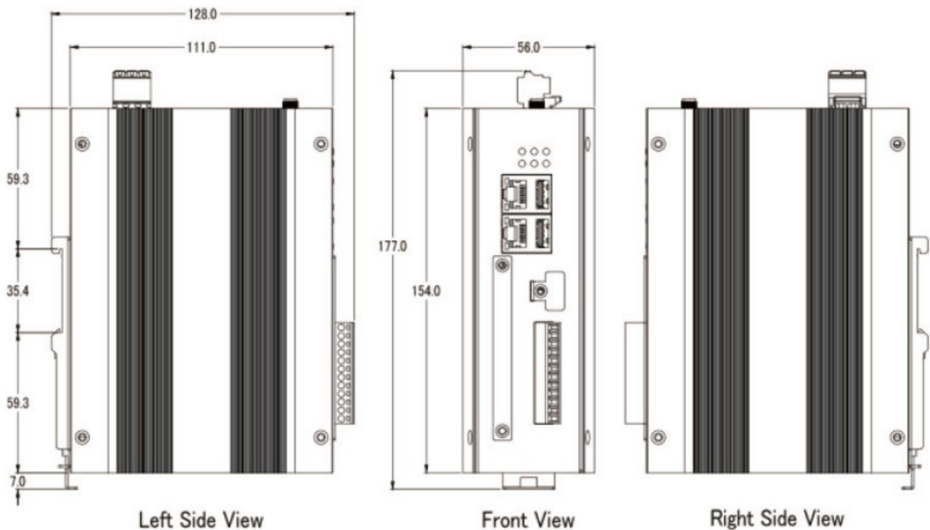
圖 1-8 BRK-2841M 尺寸圖
