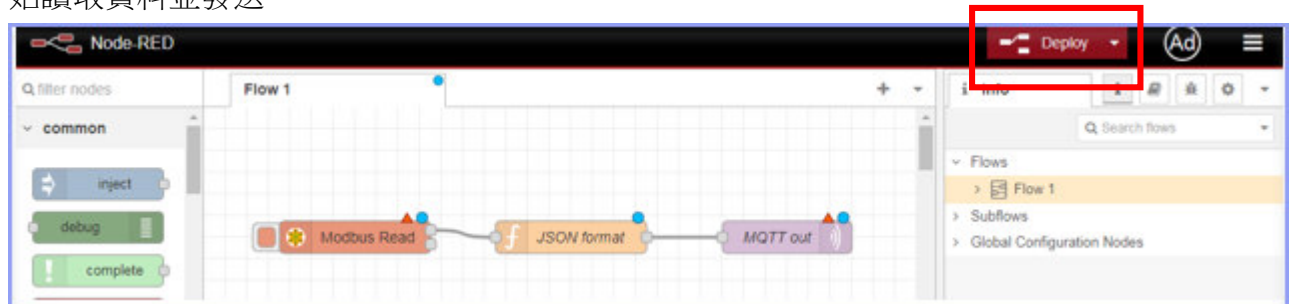
圖 6-10 部署生效
