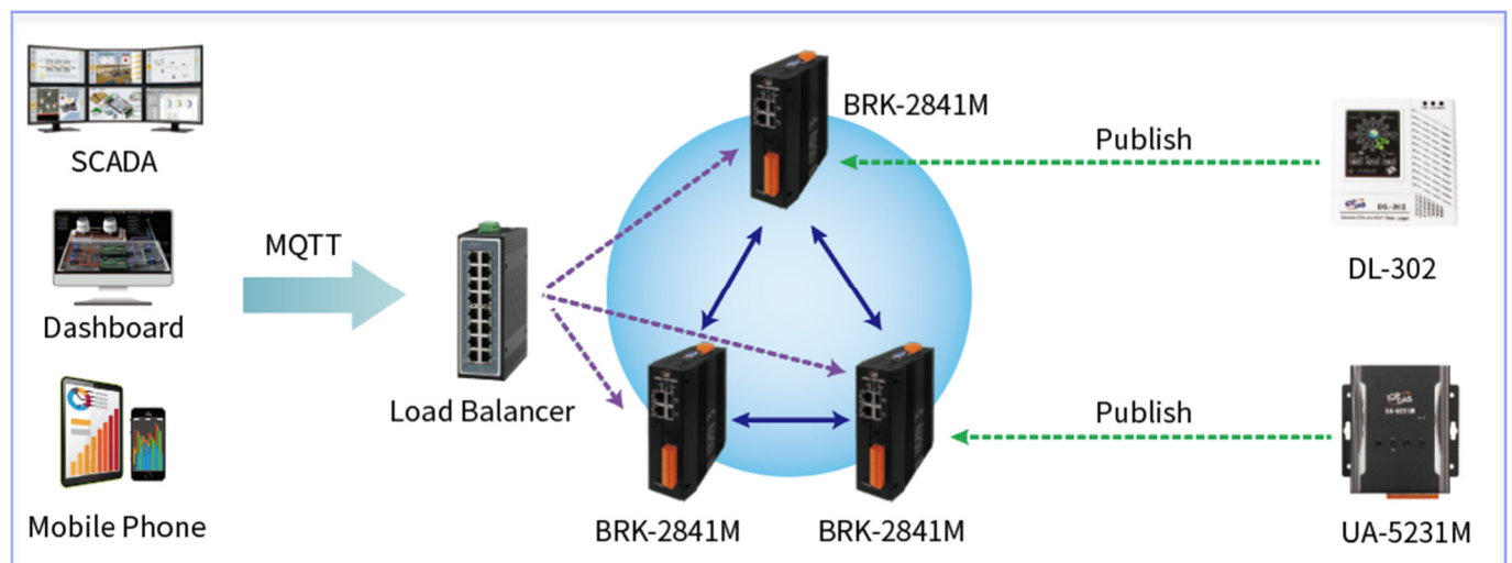
圖 4-16 叢集架構圖
