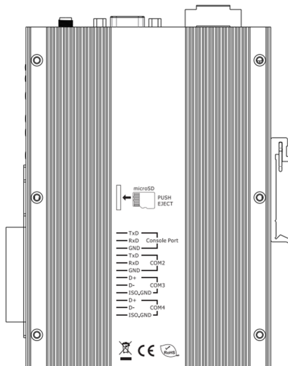
圖 1-7 BRK-2841M 機構圖(2)
