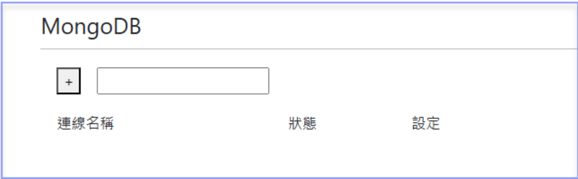
圖 4-31 MQTT 轉 MongoDB (1)
