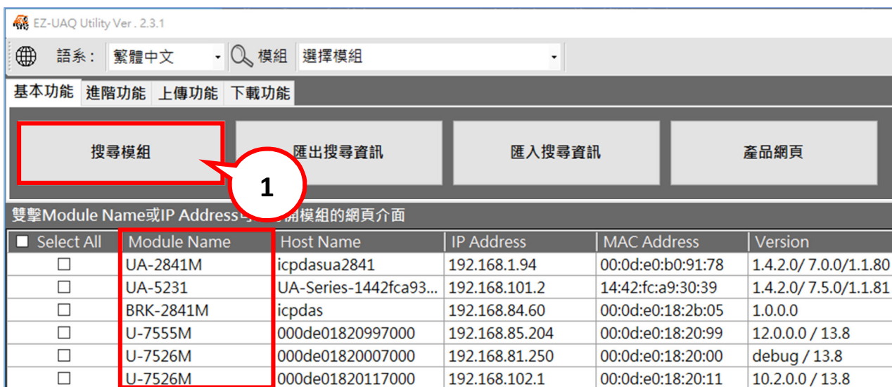
圖 2-11 搜尋模組
