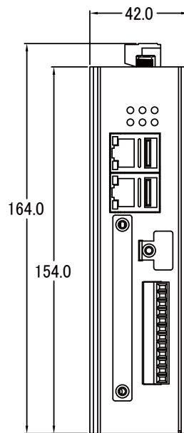
前視圖
