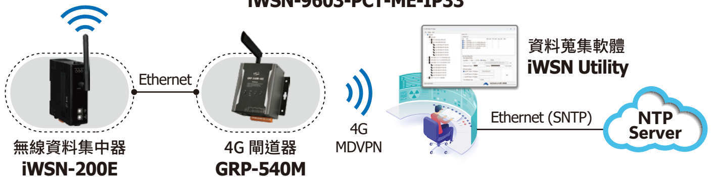
三相電力資訊量測模組 iWSN-9603-PCT-ME-IP33
