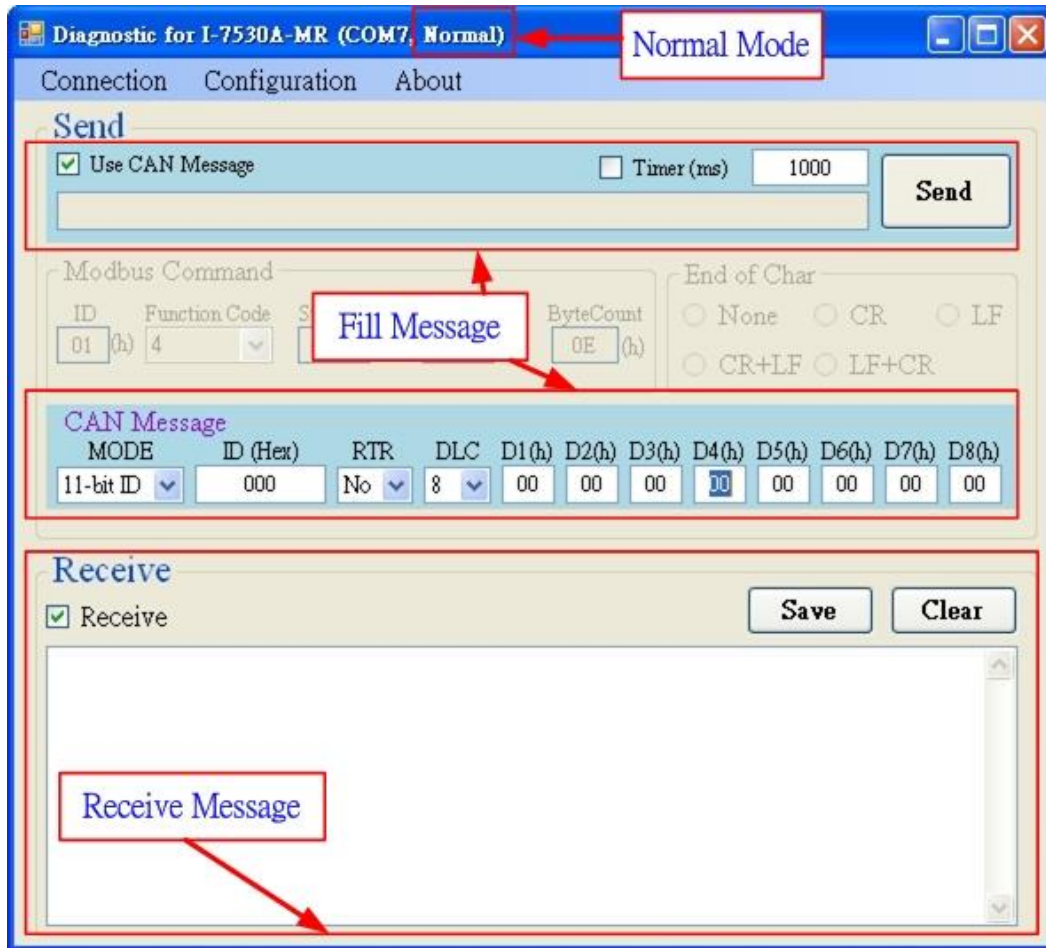
圖 3-31: 工具軟體在一般模式的有效顯示區域
