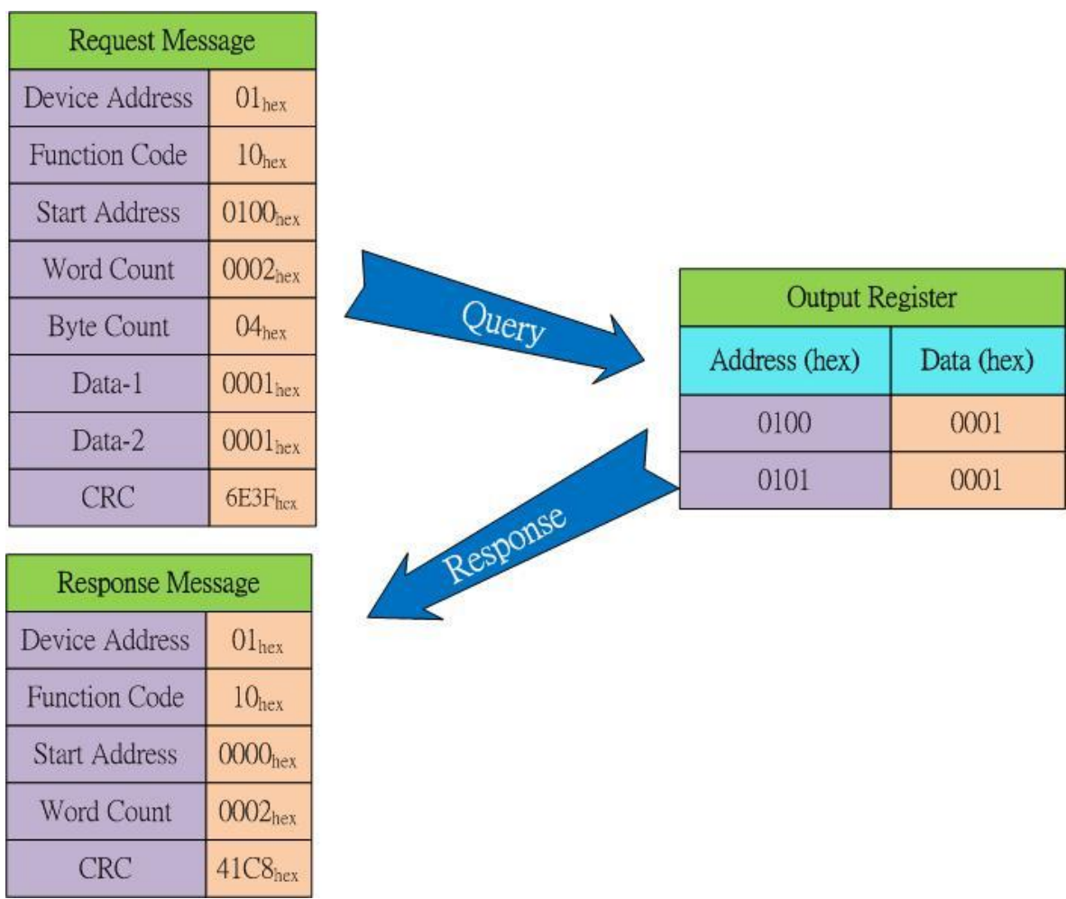
圖 5-8: 使用 Modbus 命令去重啟模組
