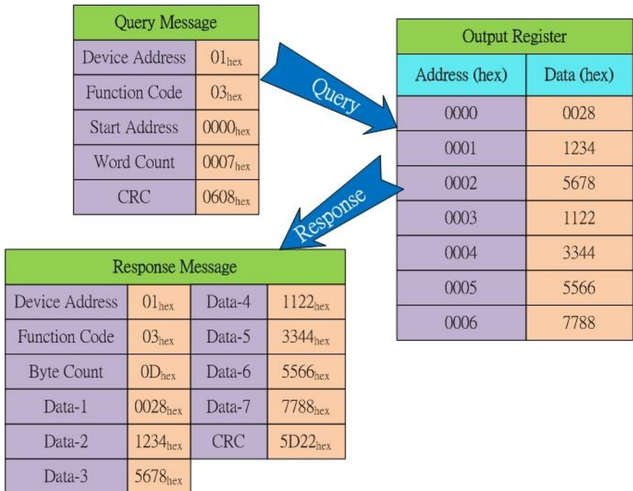
圖 5-6: 使用 Modbus RTU 命令(功能碼 03 hex) 去讀取 CAN 訊息的傳輸格式
