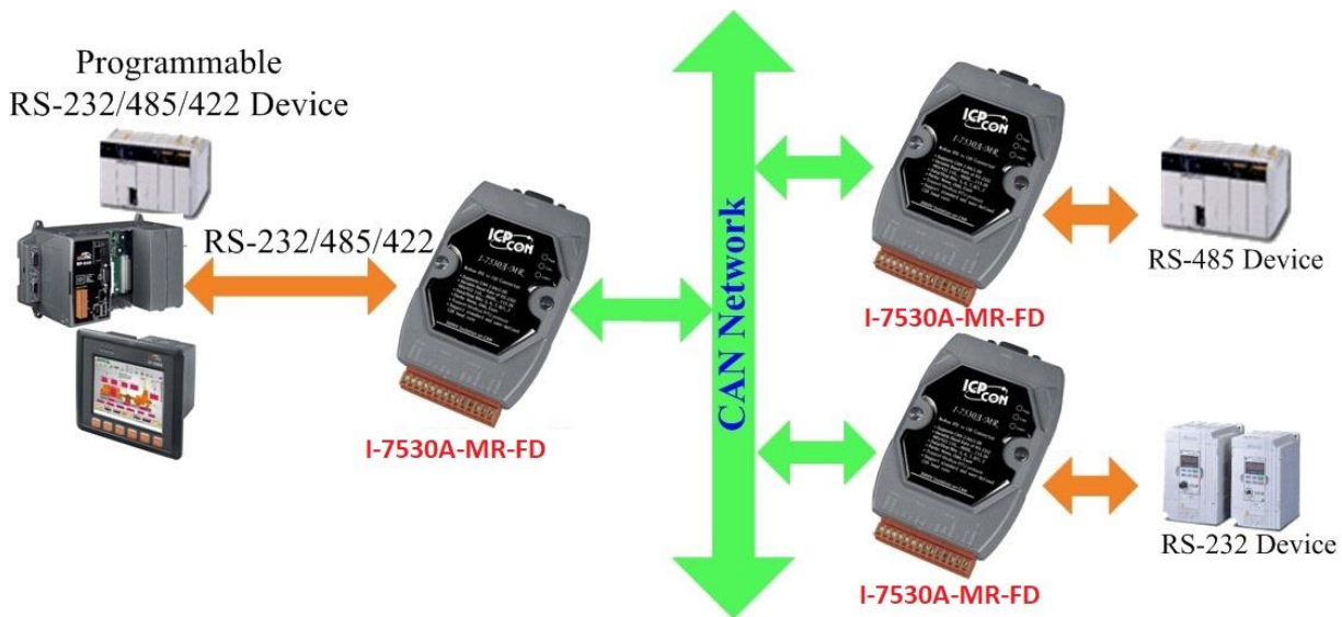
圖 1-2: Pair-connection 模式的應用架構
