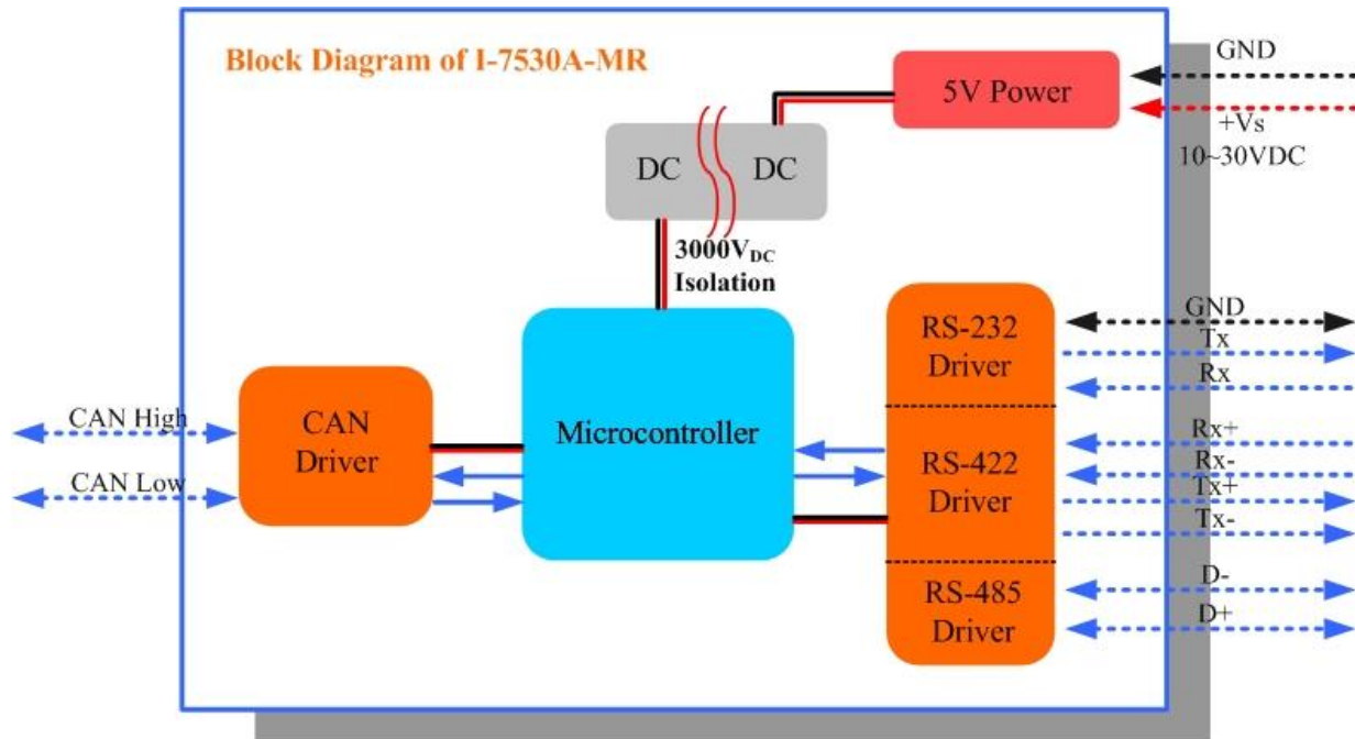
圖 2-2: I-7530A-MR-FD 的硬體方塊圖
