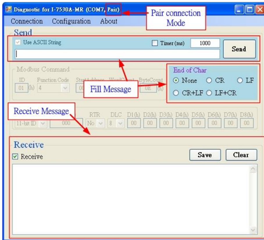
圖 3-34: 工具軟體在 Pair-connection 模式的有效顯示區域
