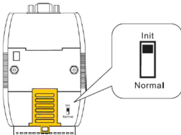
圖 2-12: I-7530A-MR-FD 的設定開關設在 Init 位置
