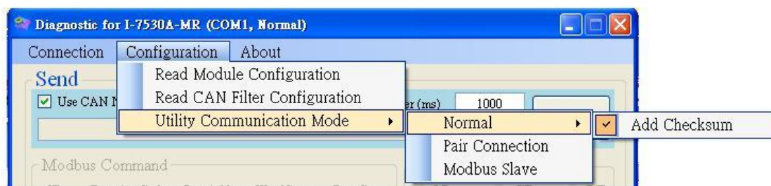
圖 3-32: 在工具中啟動 checksum 功能
