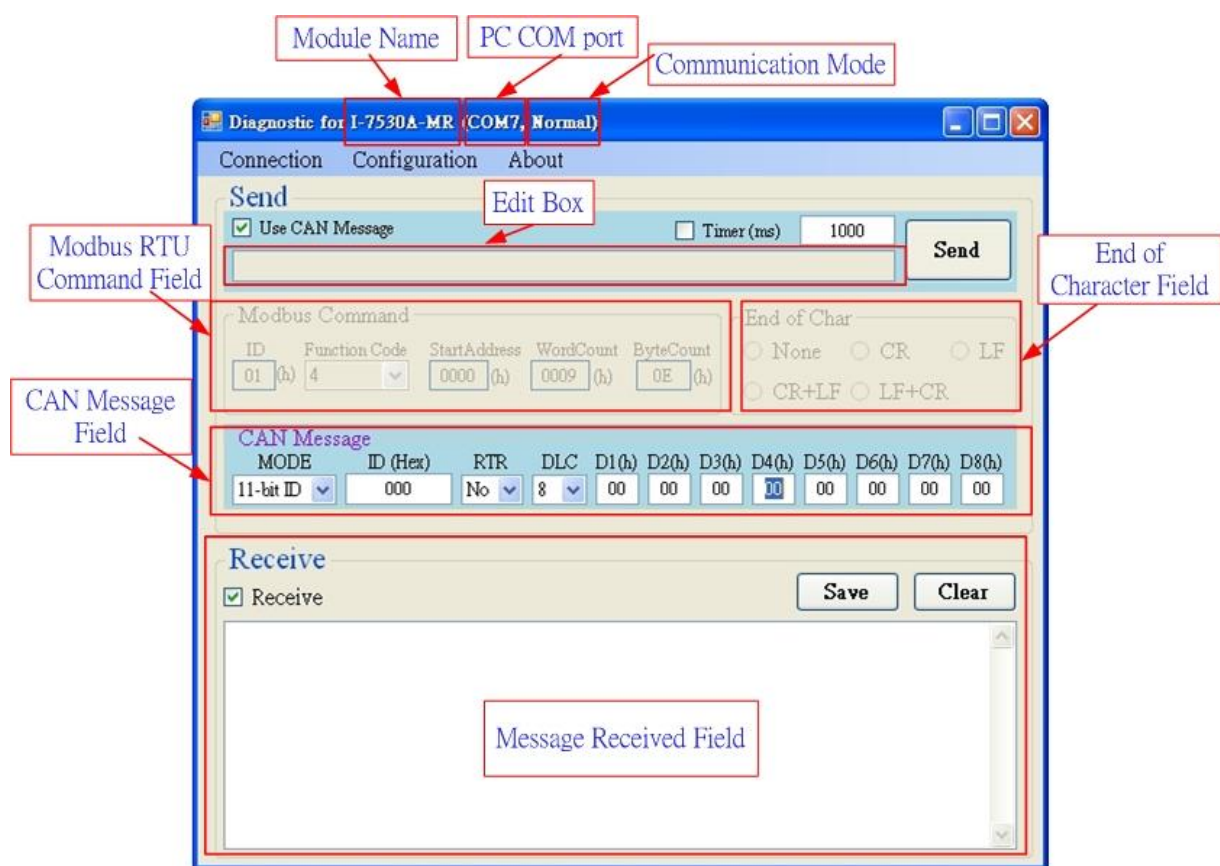
圖 3-29:診斷表的說明
