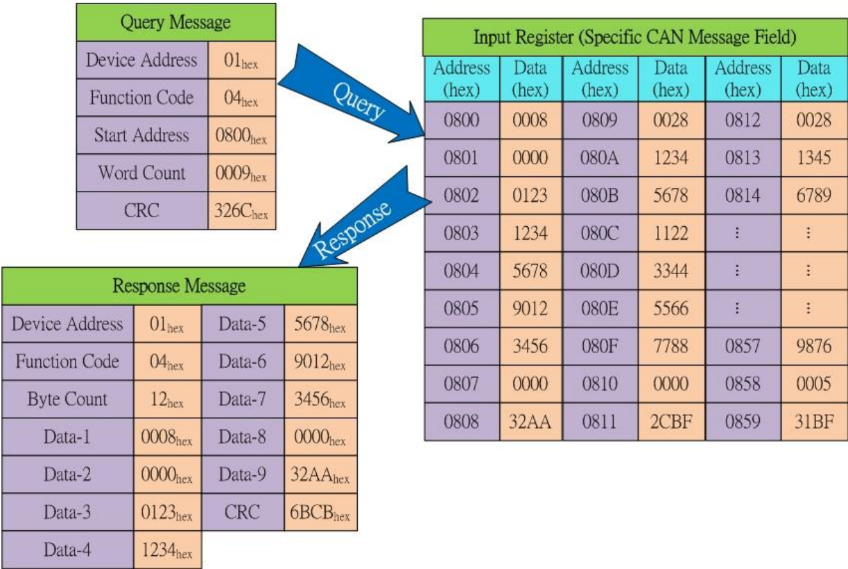
圖 5-7: 使用 Modbus 命令去讀取特定的 CAN 訊息
