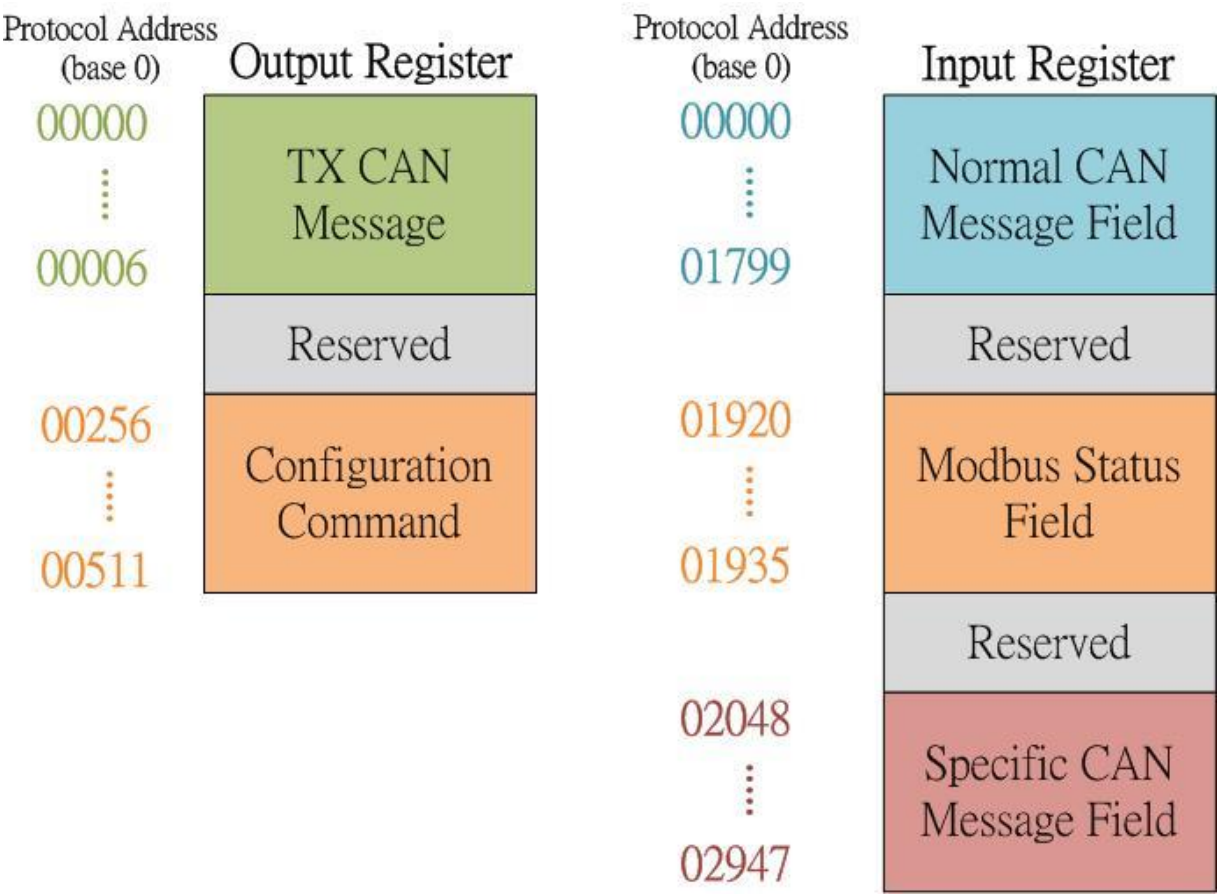
圖 5-2: 在 I-7530A-MR-FD 中，一般 CAN 訊息輸入暫存器和輸出暫存器的定義位址
