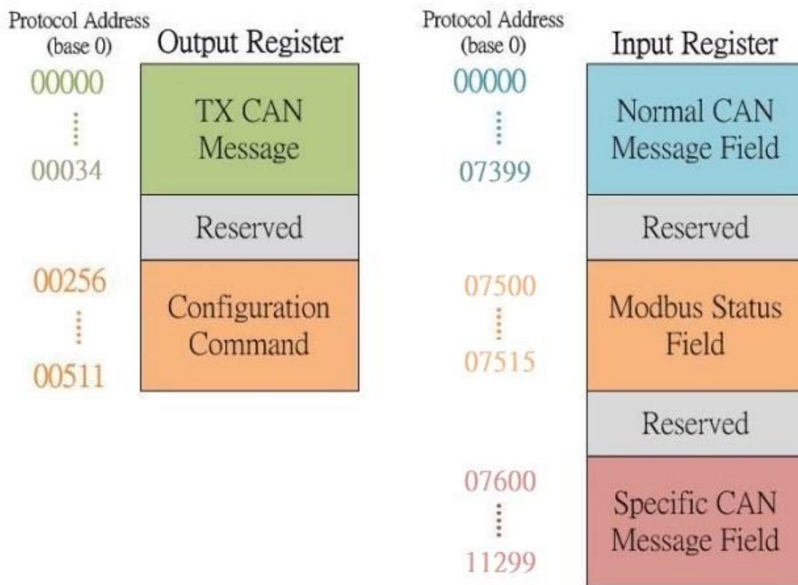
圖 5-3: 在 I-7530A-MR-FD 中，CANFD 訊息輸入暫存器和輸出暫存器的定義位址
