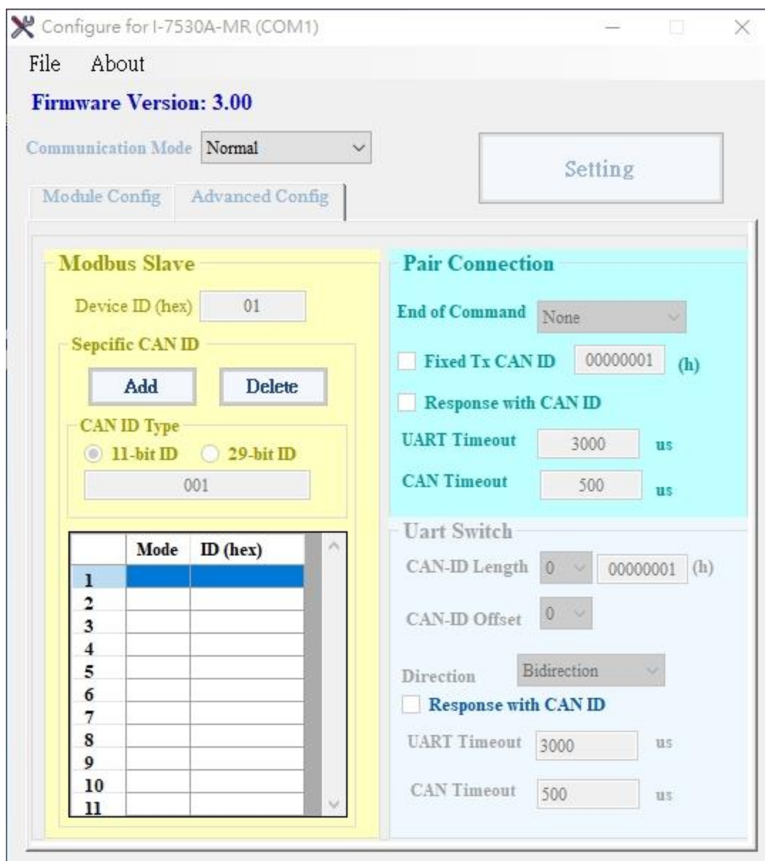
圖 3-9: I-7530A-MR-FD 模組設定格式(Slave & Pair connection & Uart Switch Mode)
