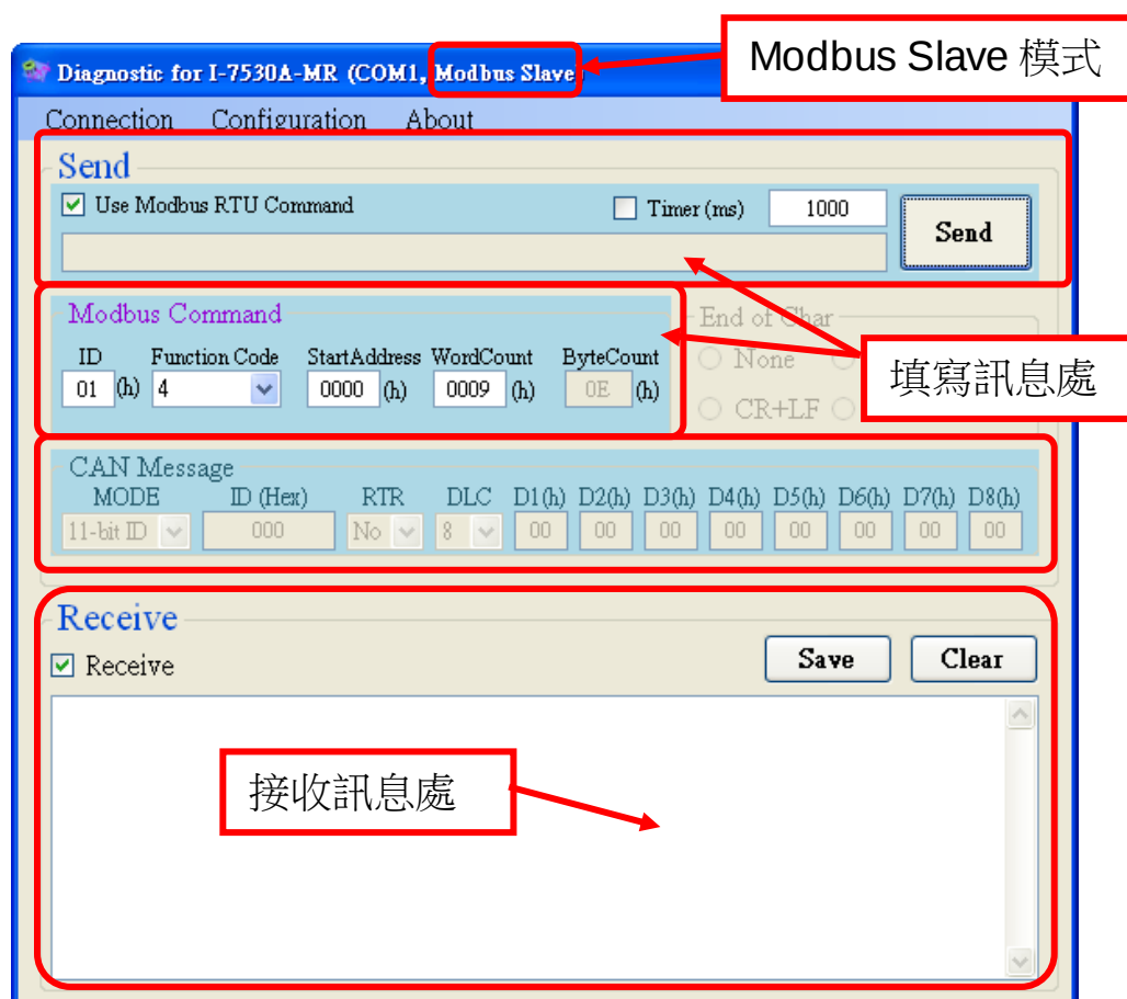
圖 3-36: 工具軟體在 Modbus Slave 模式的有效顯示區域
