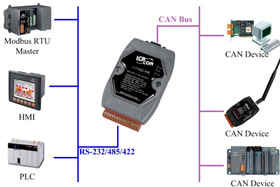
圖 1-1: Modbus Slave 模式的應用架構.
