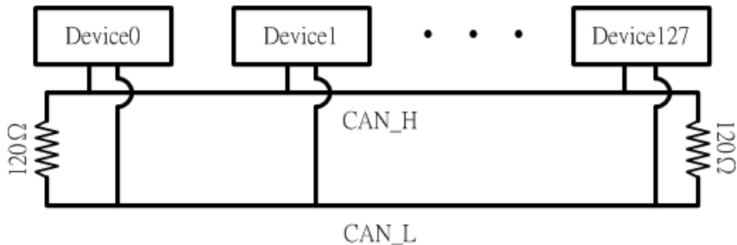
圖 2-8: 終端電阻
