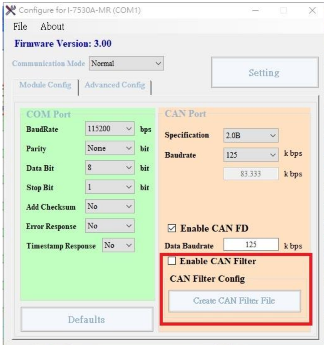
圖 3-15: CAN 過濾器的設定
