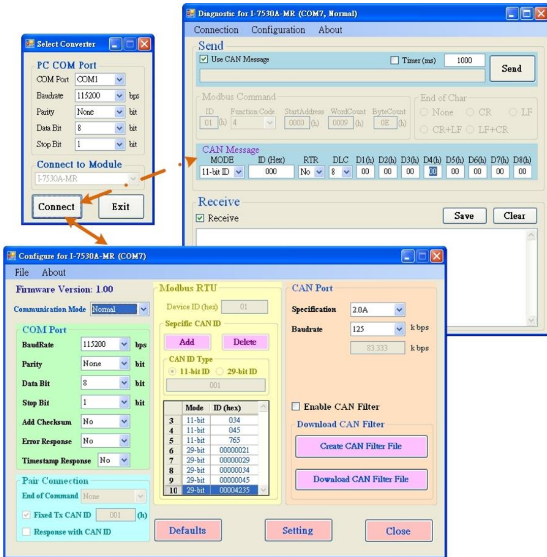
圖 3-1: UART2CAN 工具軟體設定與測試視窗
