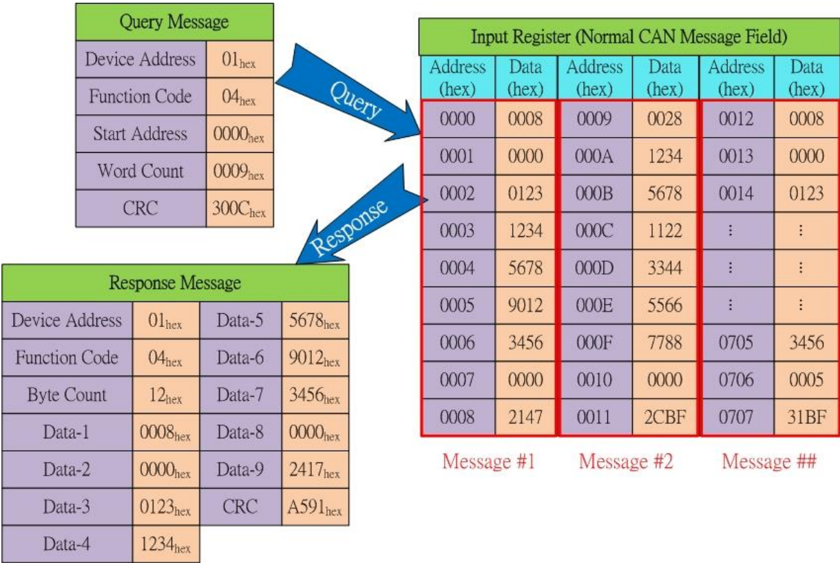
圖 5-3: 使用 Modbus 命令去讀取一個 CAN 訊息
