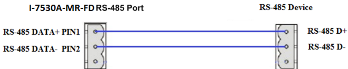
圖 2-7: RS-485 接線
