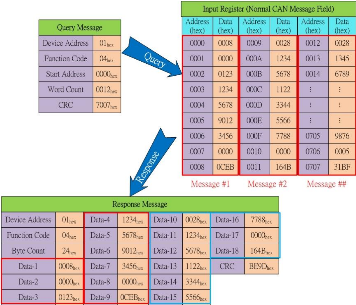
圖 5-4: 使用 Modbus Command 去讀取兩個 CAN 訊息
