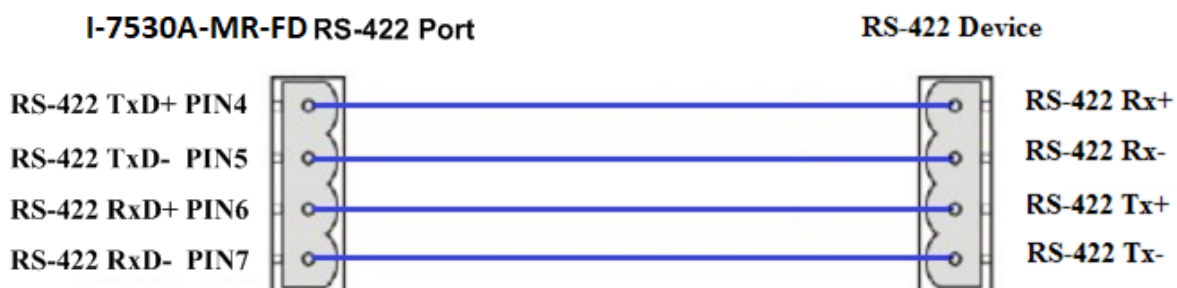
圖 2-6: RS-422 接線
