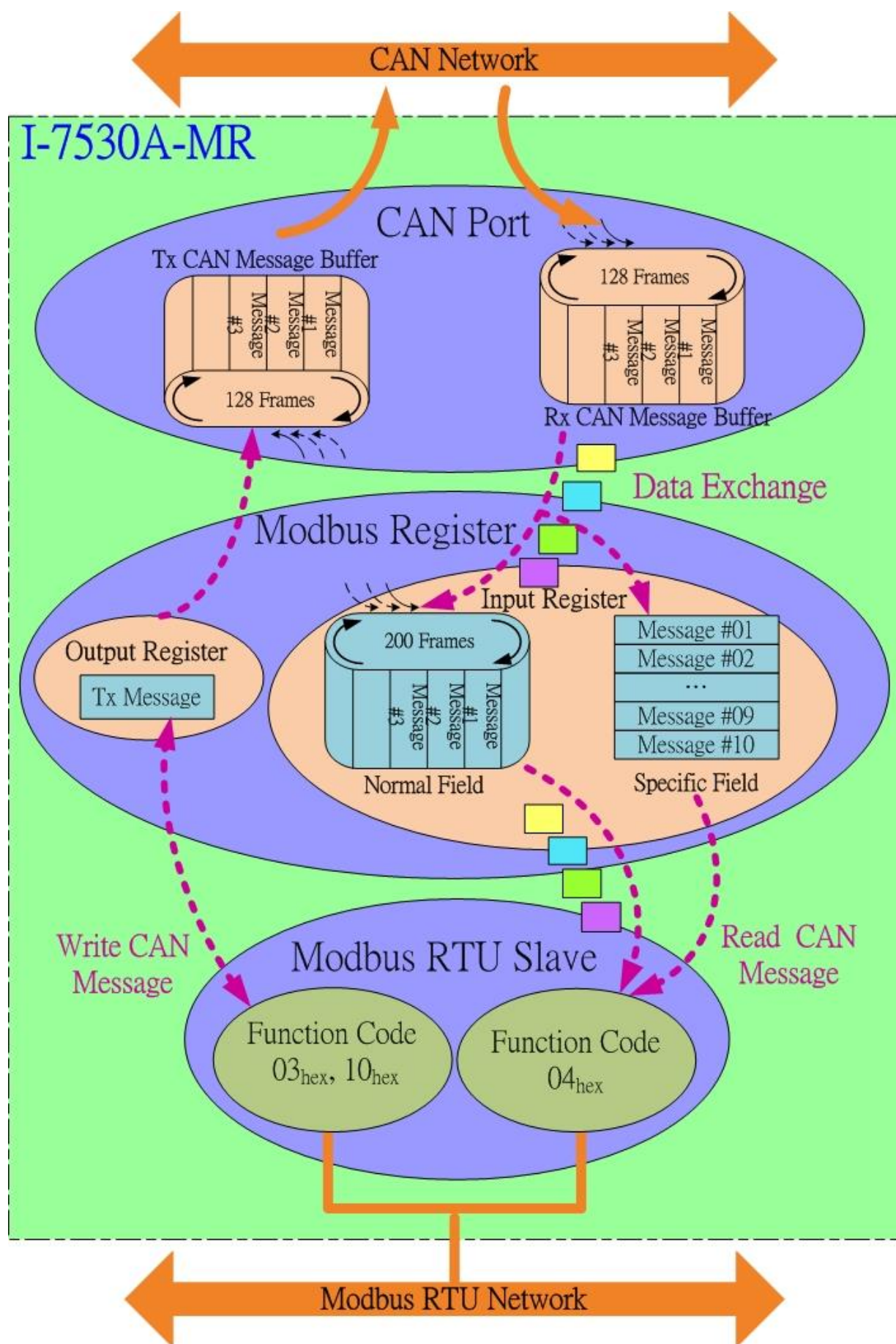
圖 5-1: Modbus 模式的結構圖
