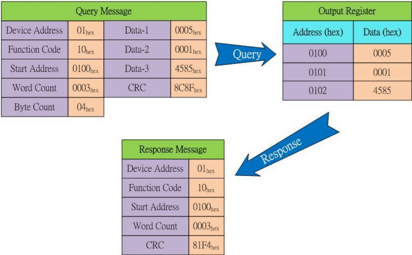
圖 5-9: 使用 Modbus 命令去變更使用者自定 CAN 總線鮑率
