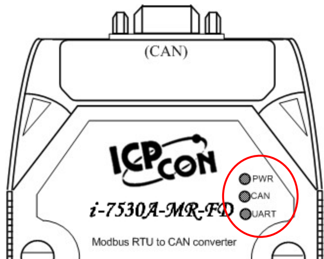
圖 2-17: I-7530A-MR-FD 的 LED 燈位置
