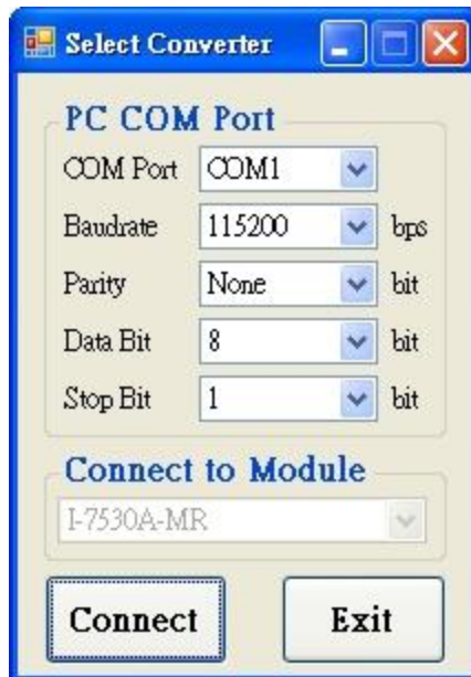
圖 3-28: 電腦 COM 端口的設定.
