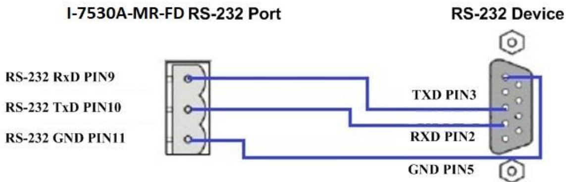
圖 2-5: RS-232 接線
