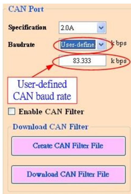
圖 6-1: 對 I-7530A-MR -FD 自訂 CAN 鮑率
