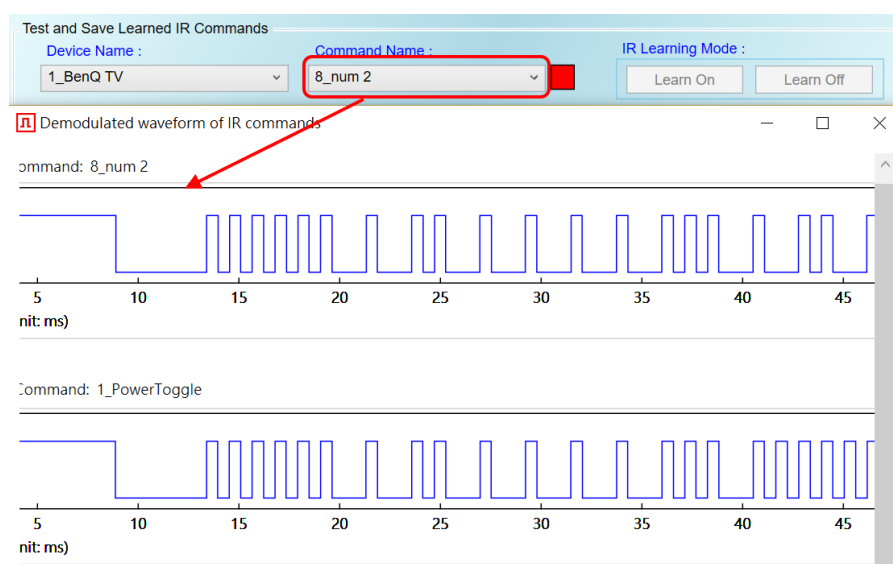
圖 3-24、前一個 IR 命令波形位於下方位置
