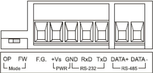
圖 2-3、IR-210 螺絲端子台
