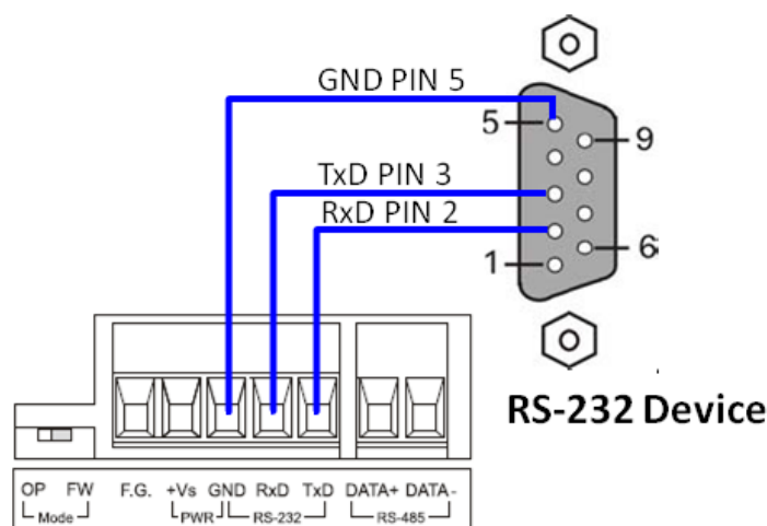
圖 2-4、RS-232 連線
