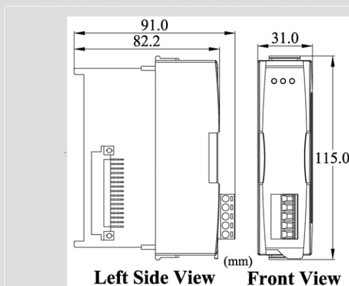
尺寸規格
