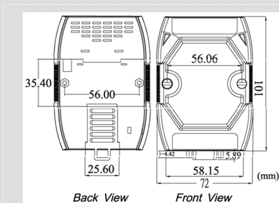
尺寸規格
