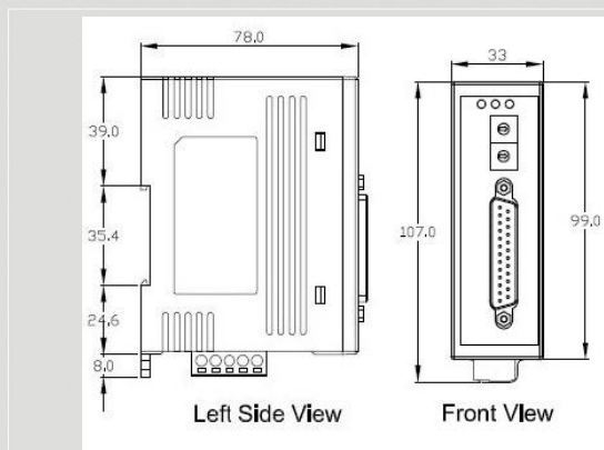
尺寸規格
