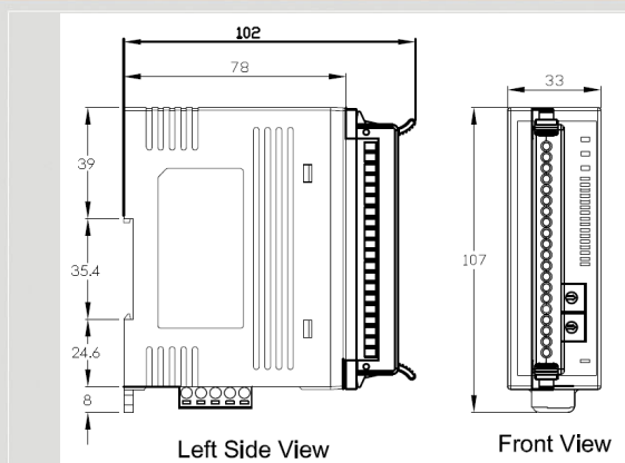
尺寸規格
