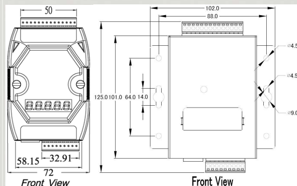
尺寸規格
