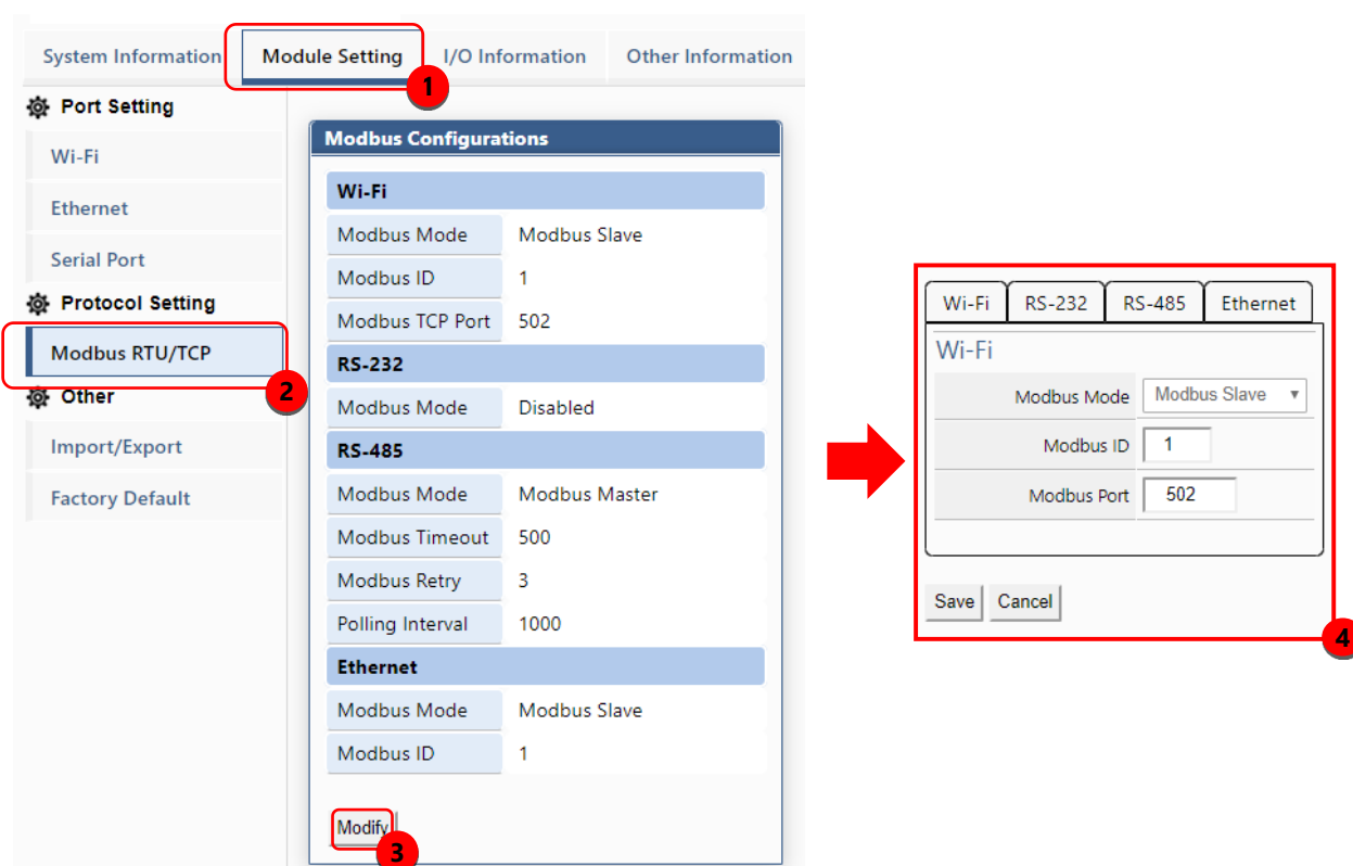
圖 2.11 Modbus RTU/TCP 通訊協議設定參數修改頁面
