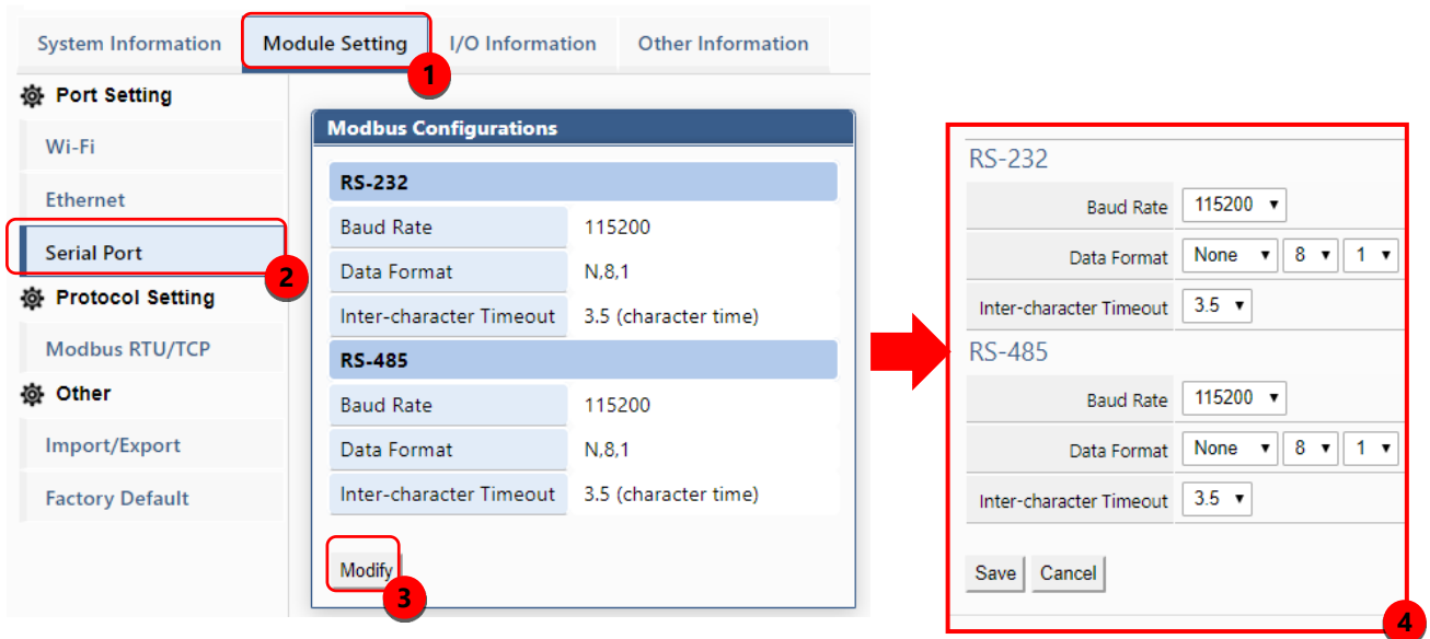
圖 2.8 當前序列埠相關設定值與參數修改頁面
