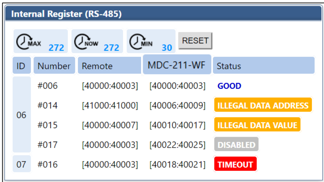
圖 5.2 Modbus 命令即時狀態範例
