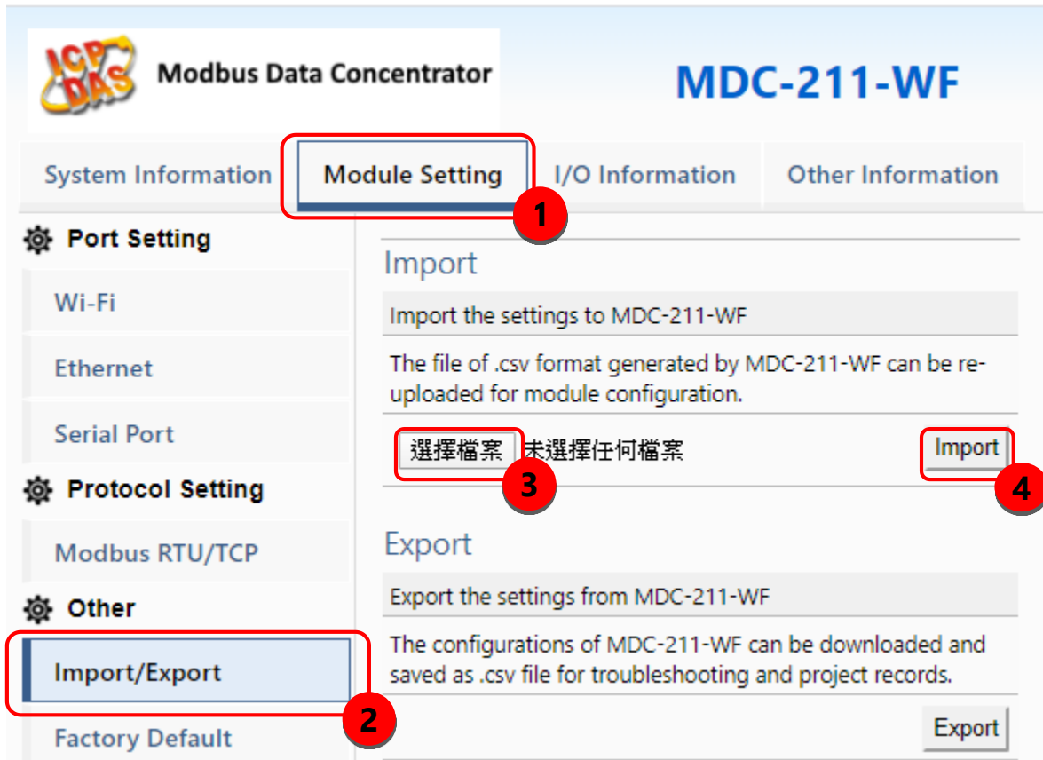
圖 3.2 模組設定參數 Import 頁面
