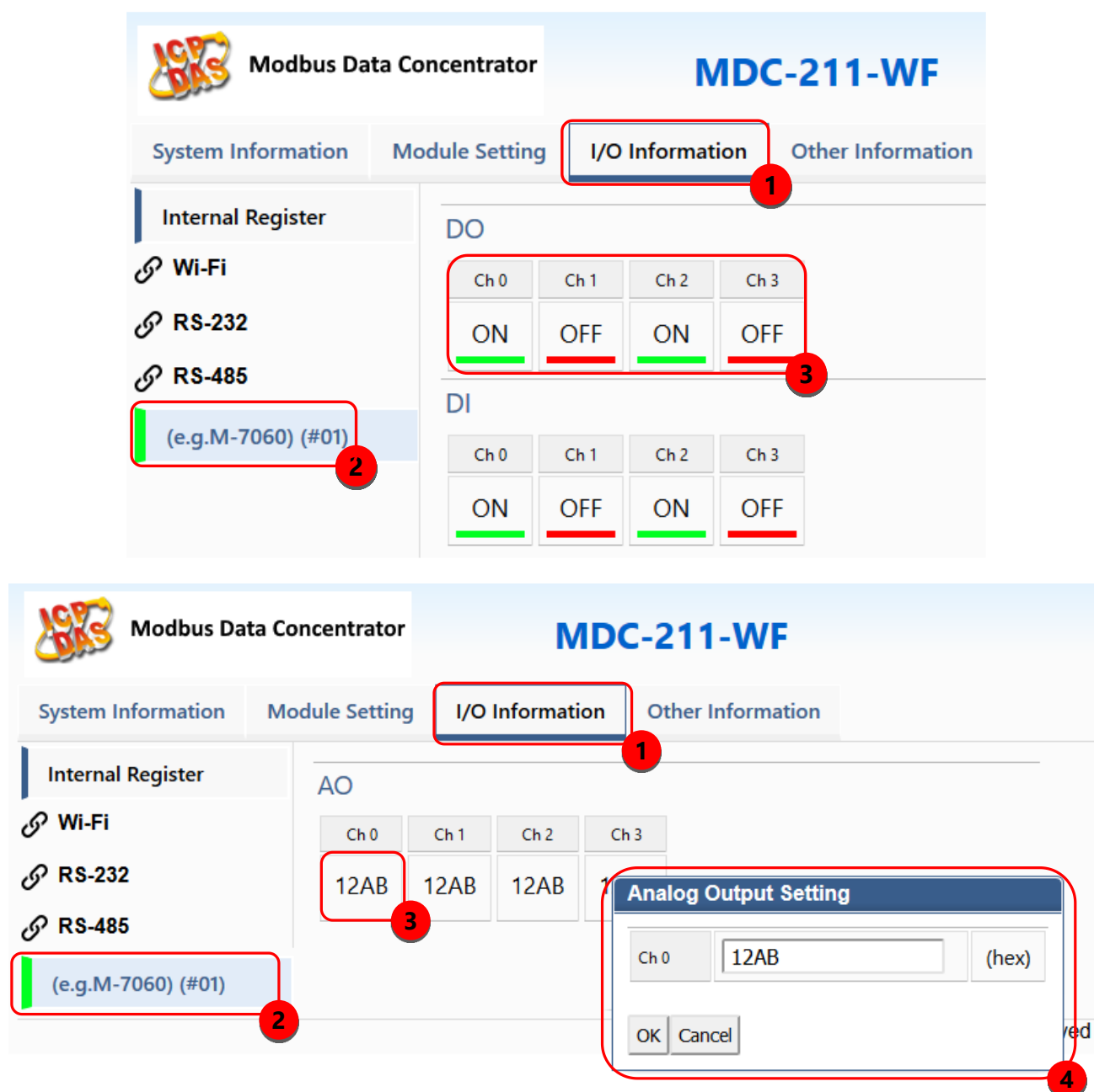
圖 2.14 Modbus I/O 資訊即時顯示頁面
