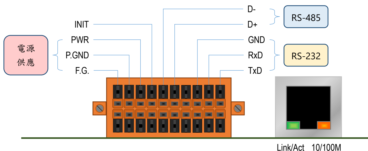
圖 2.1 MDC-211-WF 接線圖
