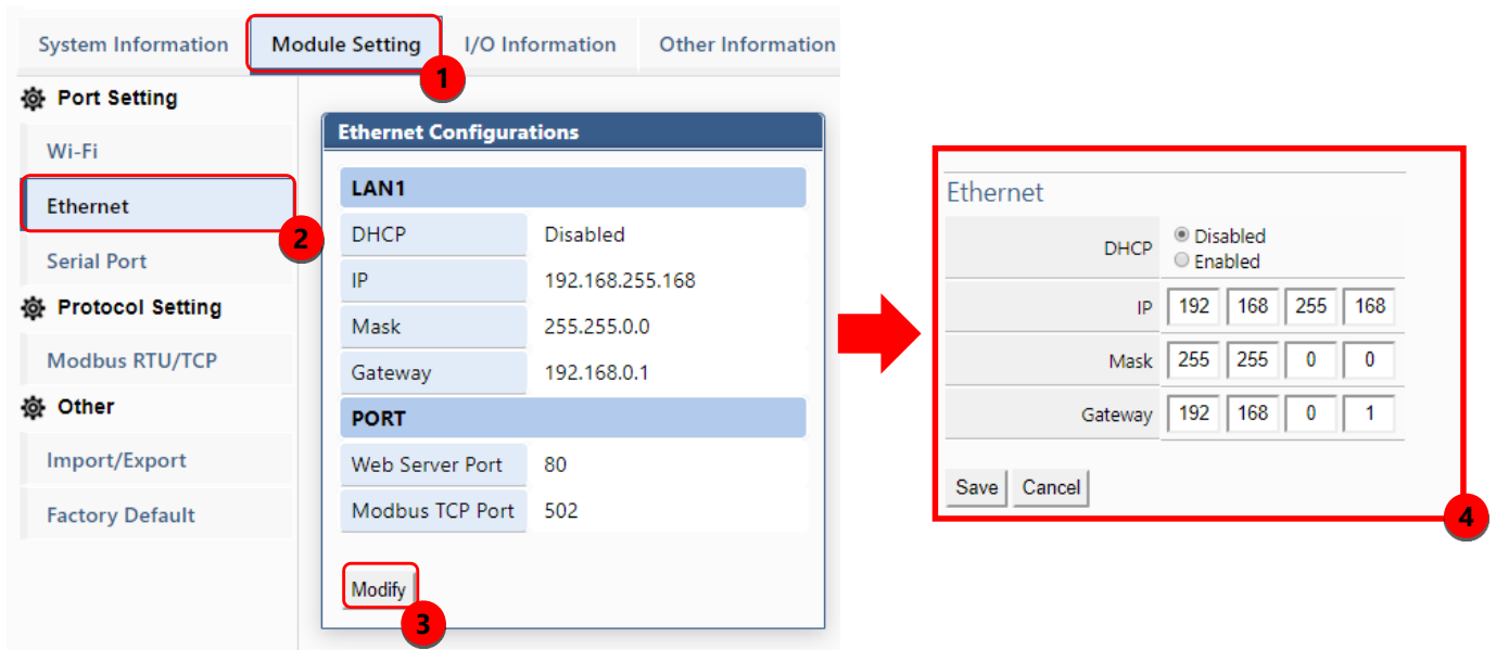
圖 2.7 當前乙太網相關設定值與參數修改頁面
