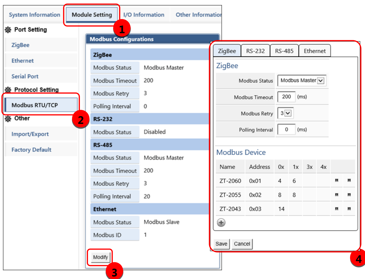
圖 2.9 當前 Modbus RTU/TCP 相關設定參數及其設定頁面
