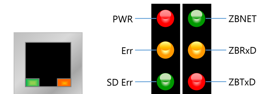
圖 6.1 LED 指示燈位置示意圖
