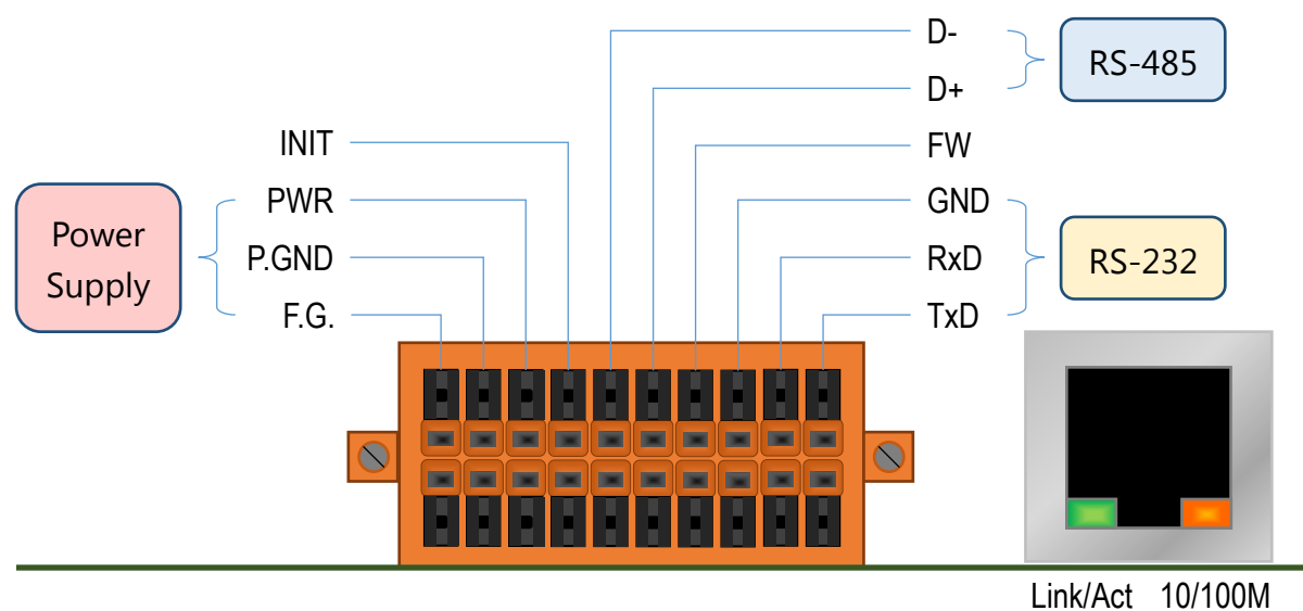
圖 2.1 MDC-211-ZT 接線圖
