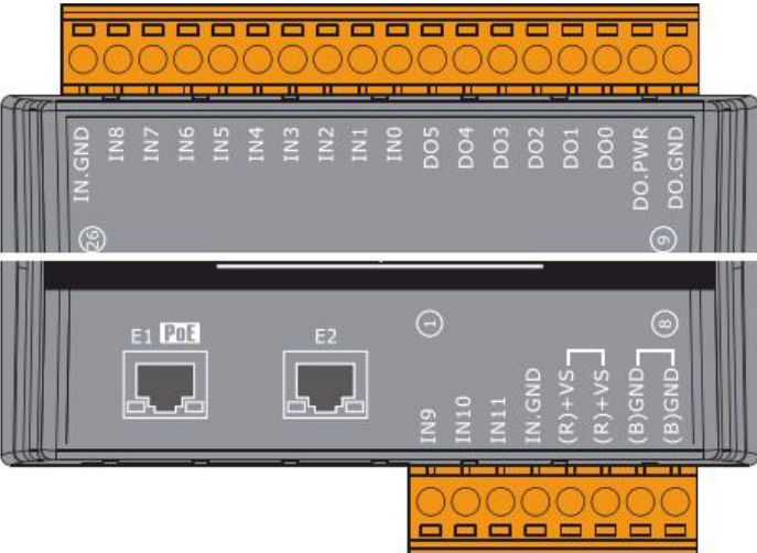
ET-7250A/PET-7250A
