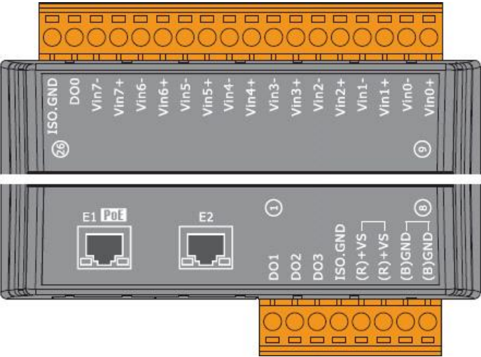
ET-7217-A5/PET-7217-A5
