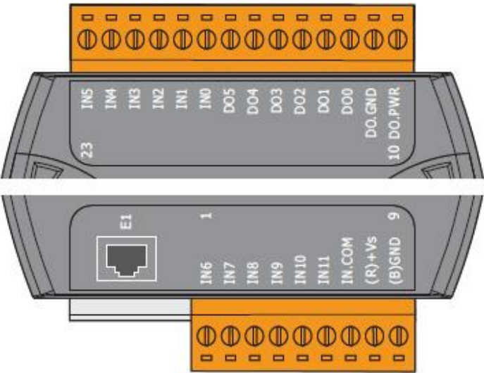
ET-7250A/PET-7250A
