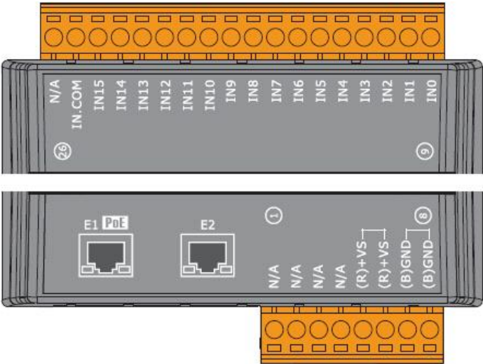
ET-7251/PET-7251
