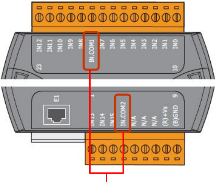
ET-7051/PET-7051
