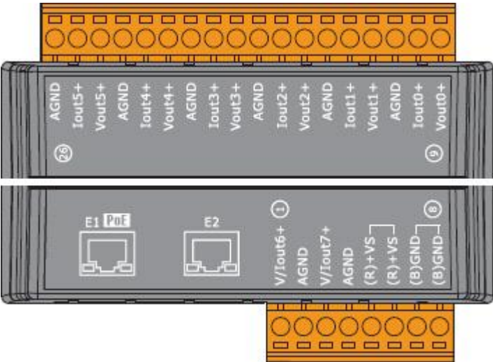
ET-7228/PET-7228
