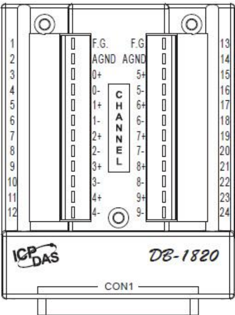
DB-1820
