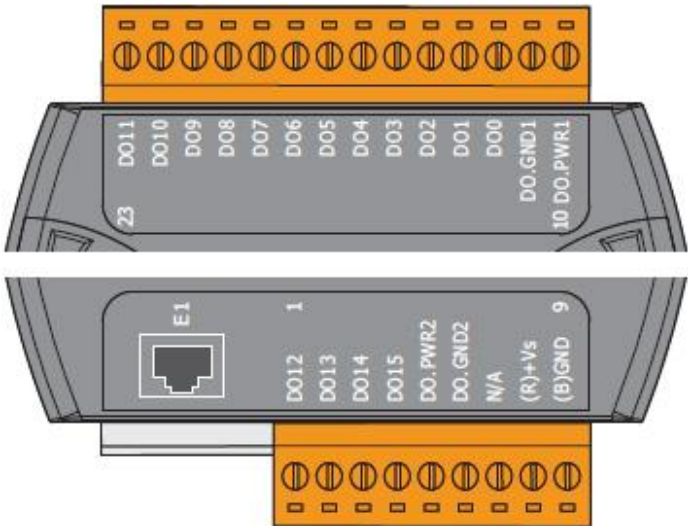
ET-7242/PET-7242
