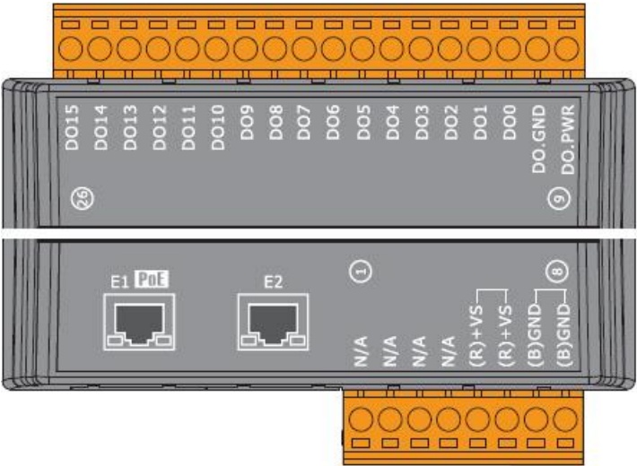
ET-7242/PET-7242
