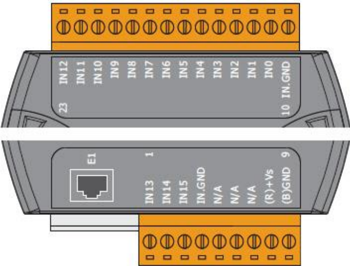
PET-7053
