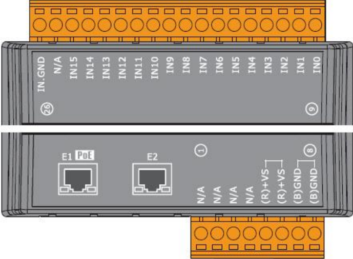
ET-7253/PET-7253
