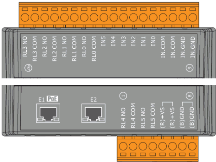
ET-7260A/PET-7260A
