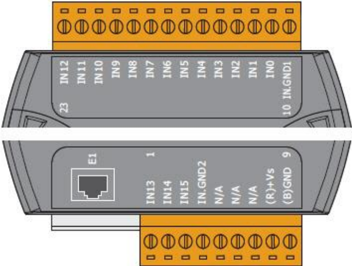
ET-7253/PET-7253
