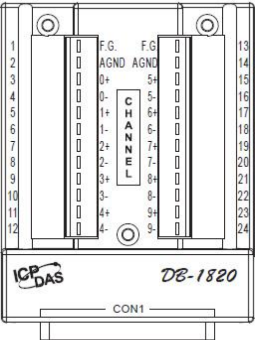
DB-1820
