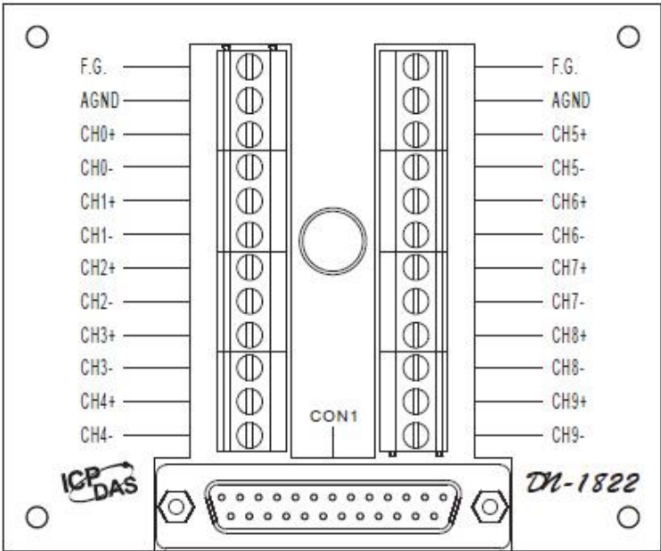
DN-1822
