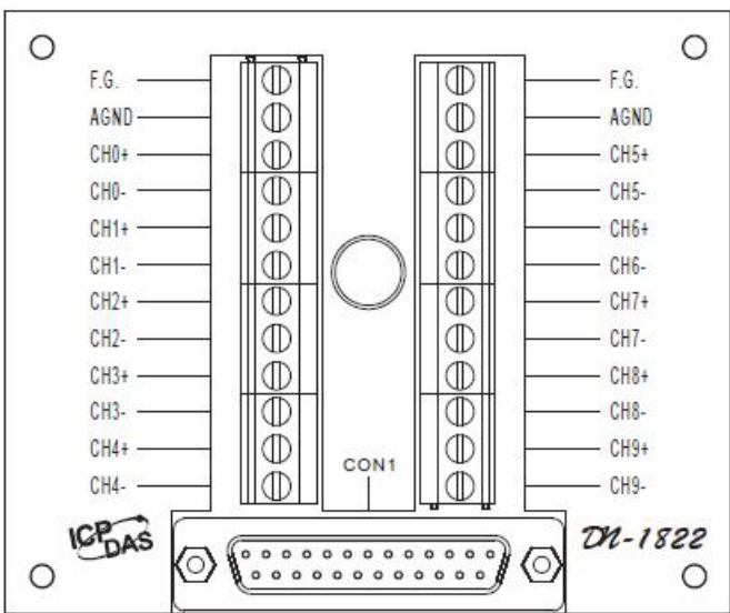
DN-1822
