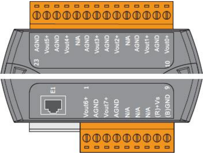
ET-7228/PET-7228
