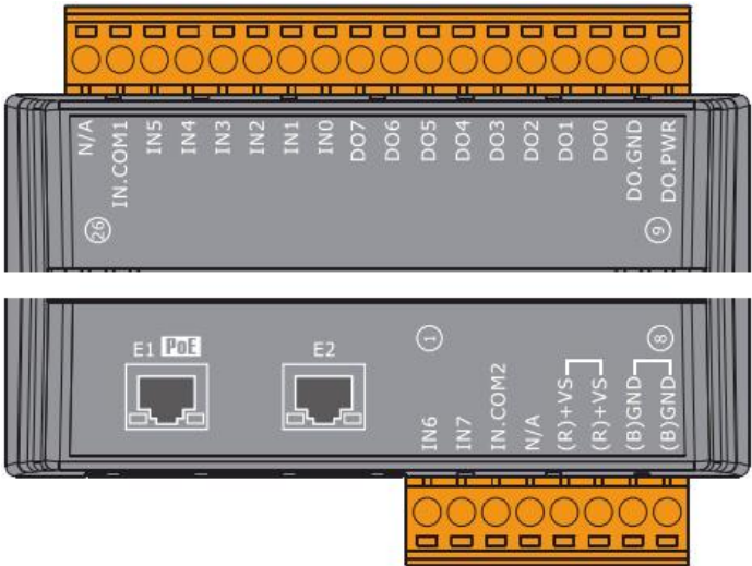
ET-7244/PET-7244
