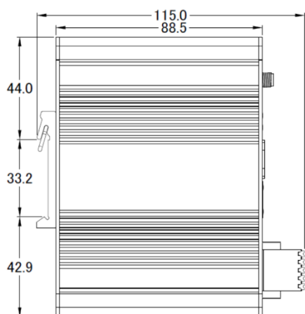
左視圖
