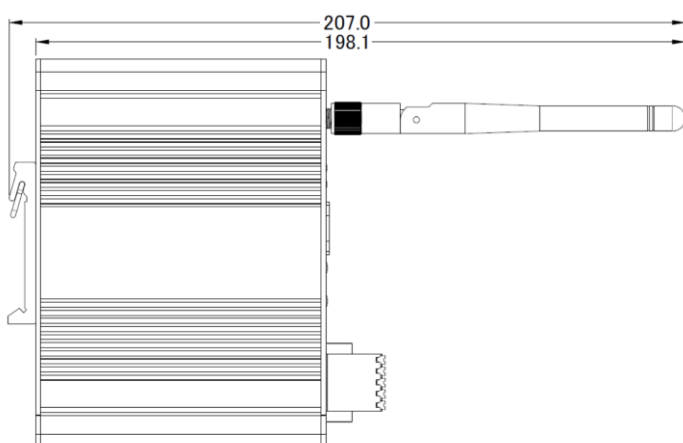
天線安裝圖 (0 度)
