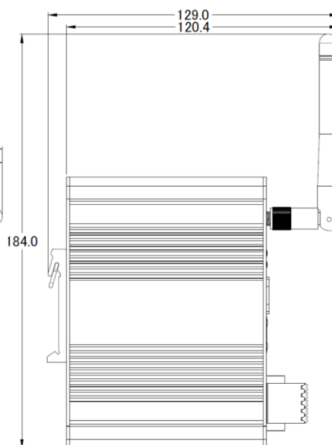
天線安裝圖 (90 度)
