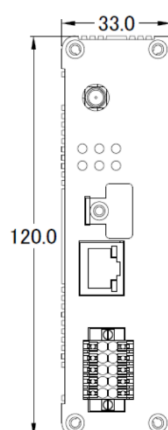
前視圖
