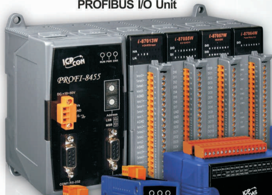
PROFIBUS I/O Unit
