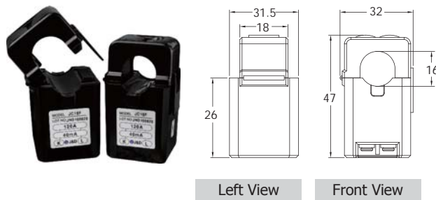
160: CTΦ16mm (100 A Max.)
