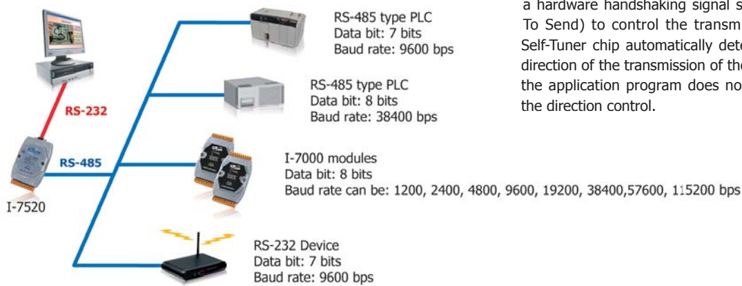
▲ I-7520
