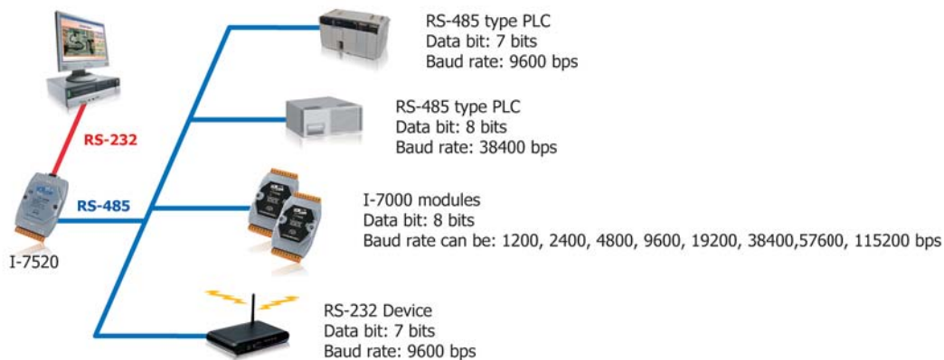
▲ I-7520
