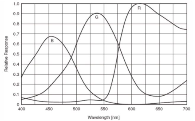
光譜感光度
