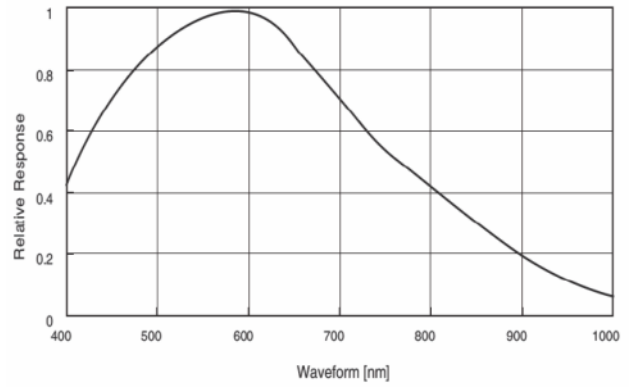
光譜感光度
