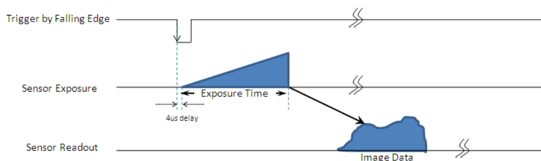
圖 1.4.10.2 下降邊緣(Falling Edge)訊號的標準觸發
