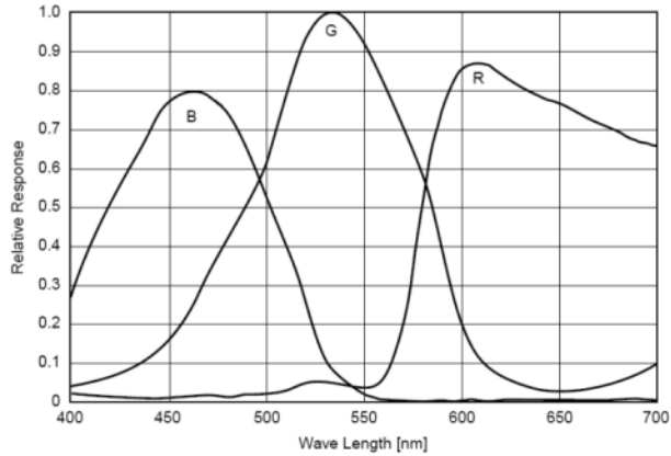
光譜感光度
