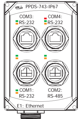
PDS-743-IP67
